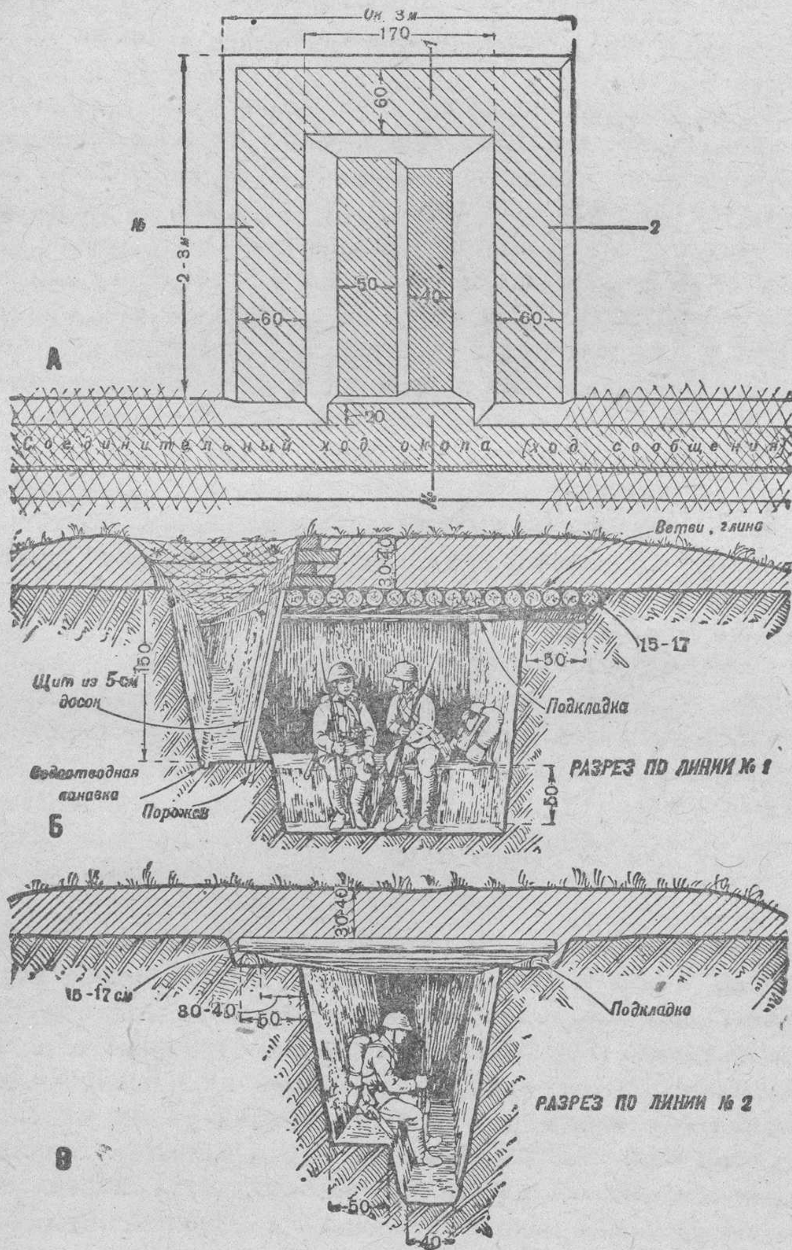
Рис. 58. Подбрустверный блиндаж:
