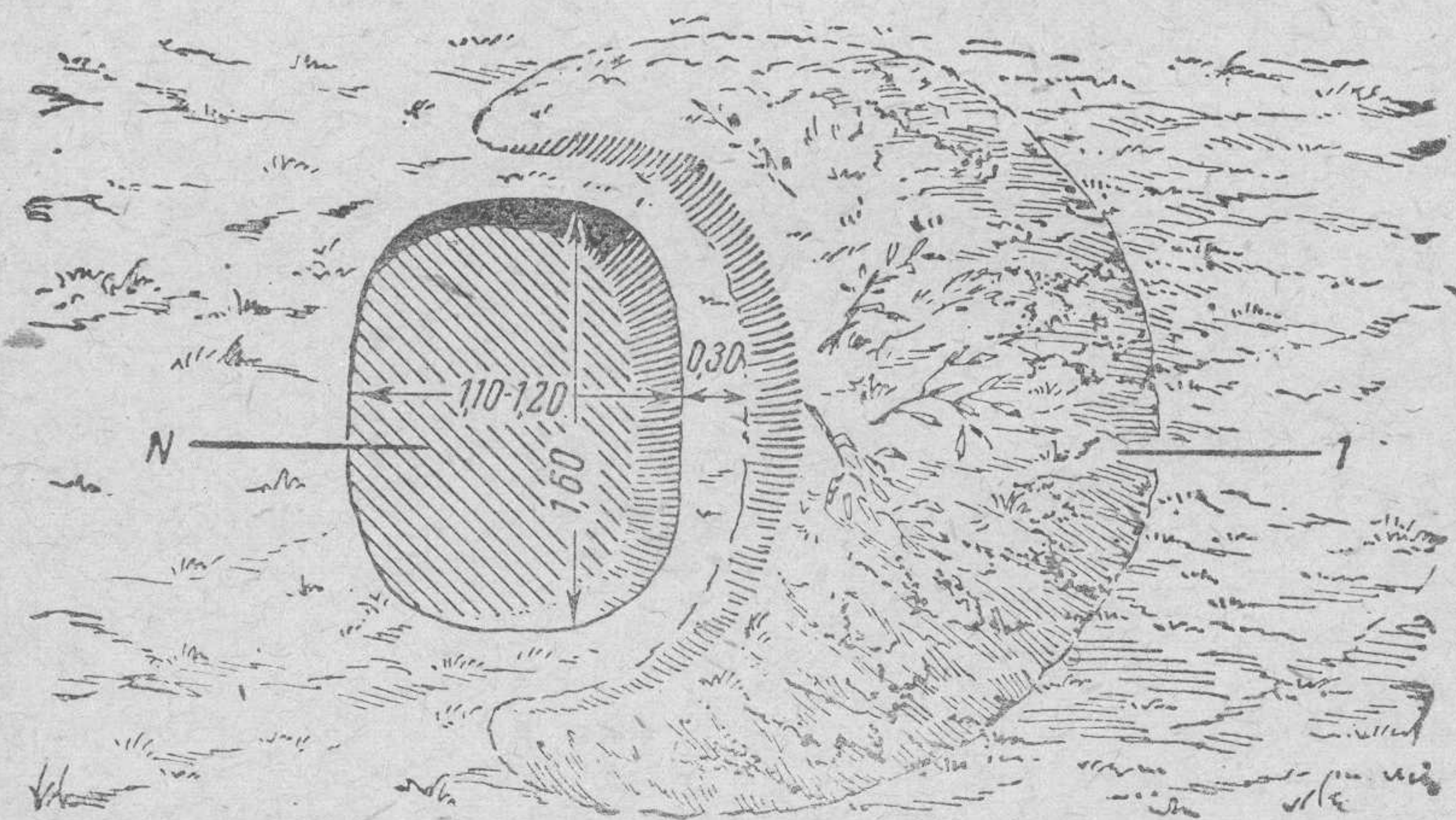
Рис. 15. Ячейка для ведения огня из противотанкового ружья Два бойца малыми лопатами отроют себе ячейку и замаскируют ее за 10 — 15 минут
