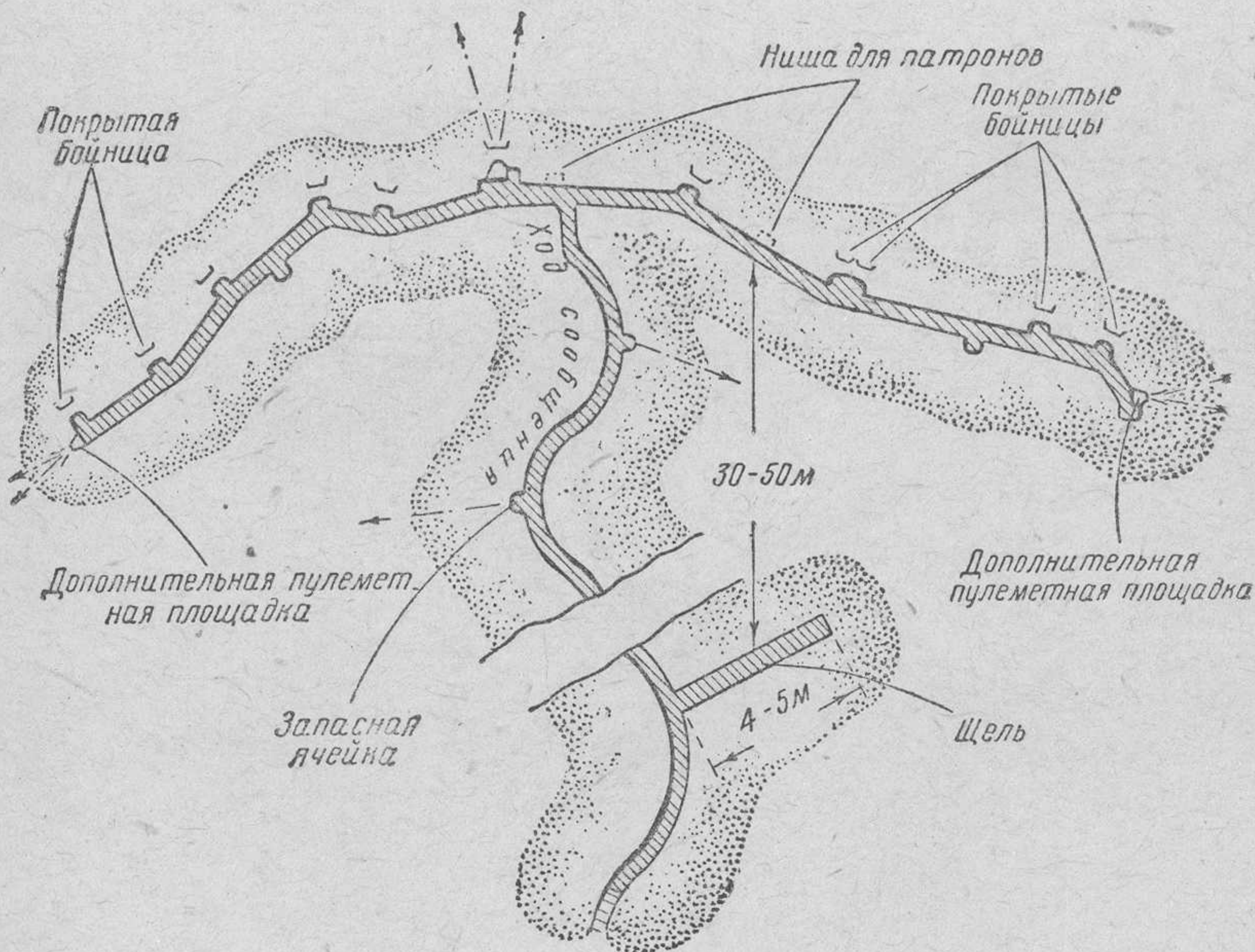
Рис. 4. Ячейковый окоп на стрелковое отделение с ходом сообщения в тыл и щелью, отрытый за одни сутки работы
