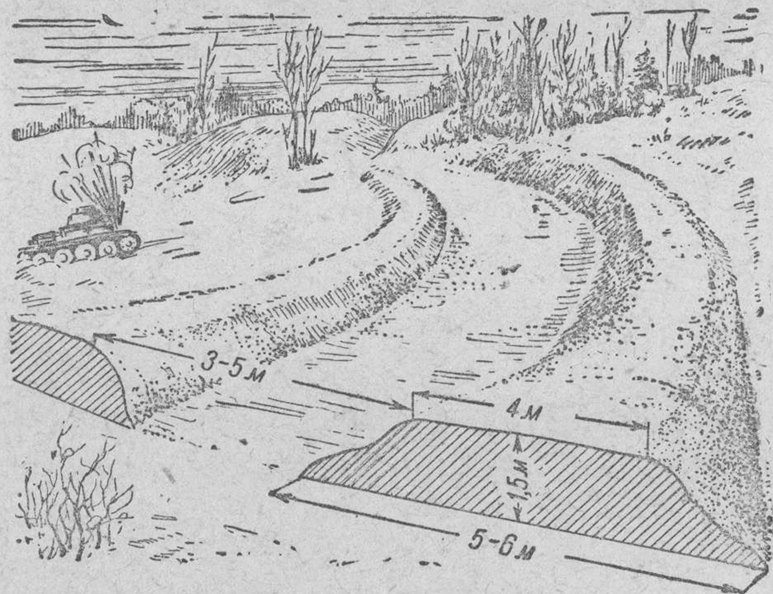
Рис. 116. Снеговые валы
