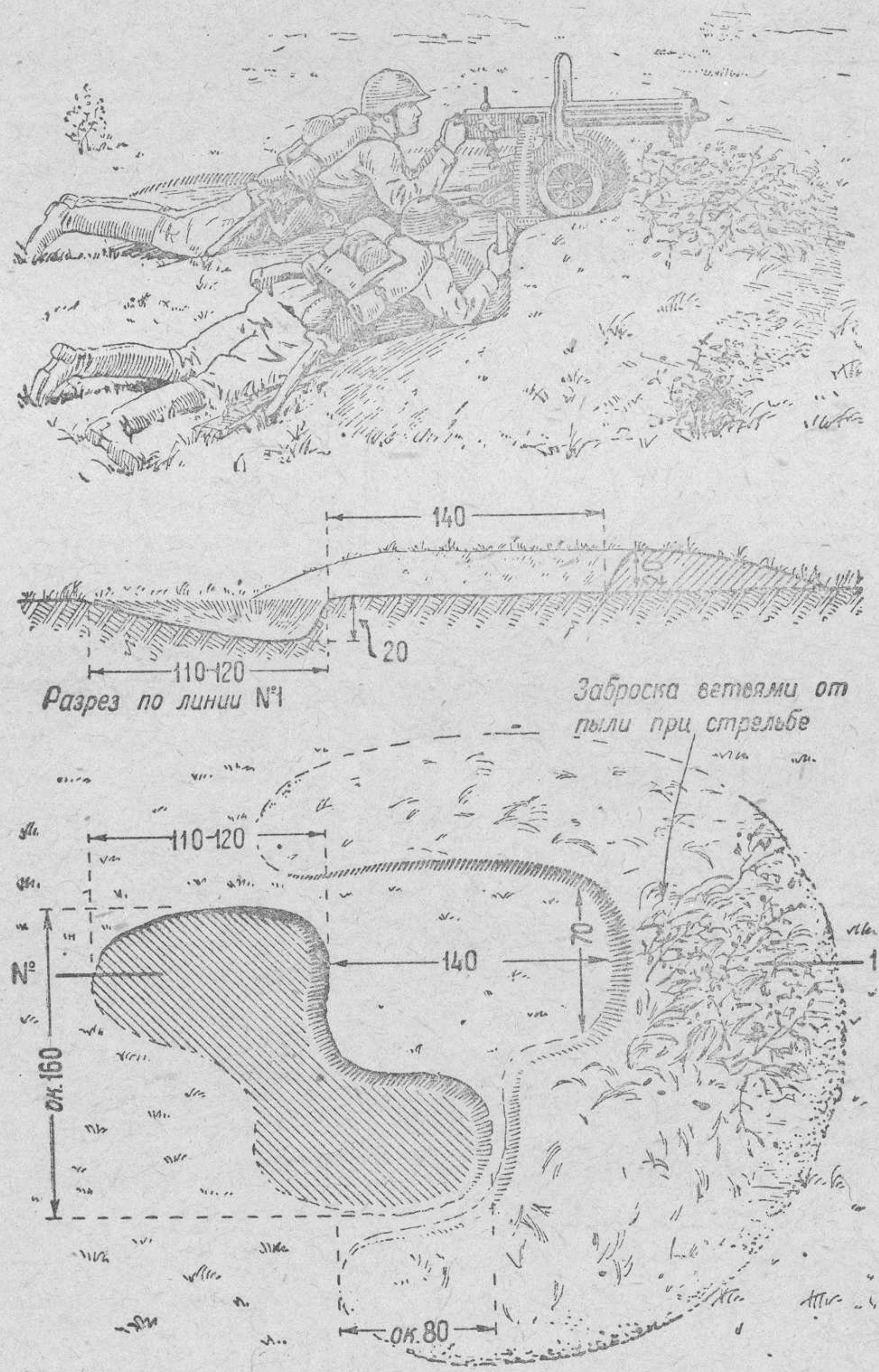
Рис. 14, А. Ячейка для ведения огня из станкового пулемета лежа Наводчик пулемета и его помощник малыми лопатами отроют ячейку и замаскируют ее за 10—15 минут
