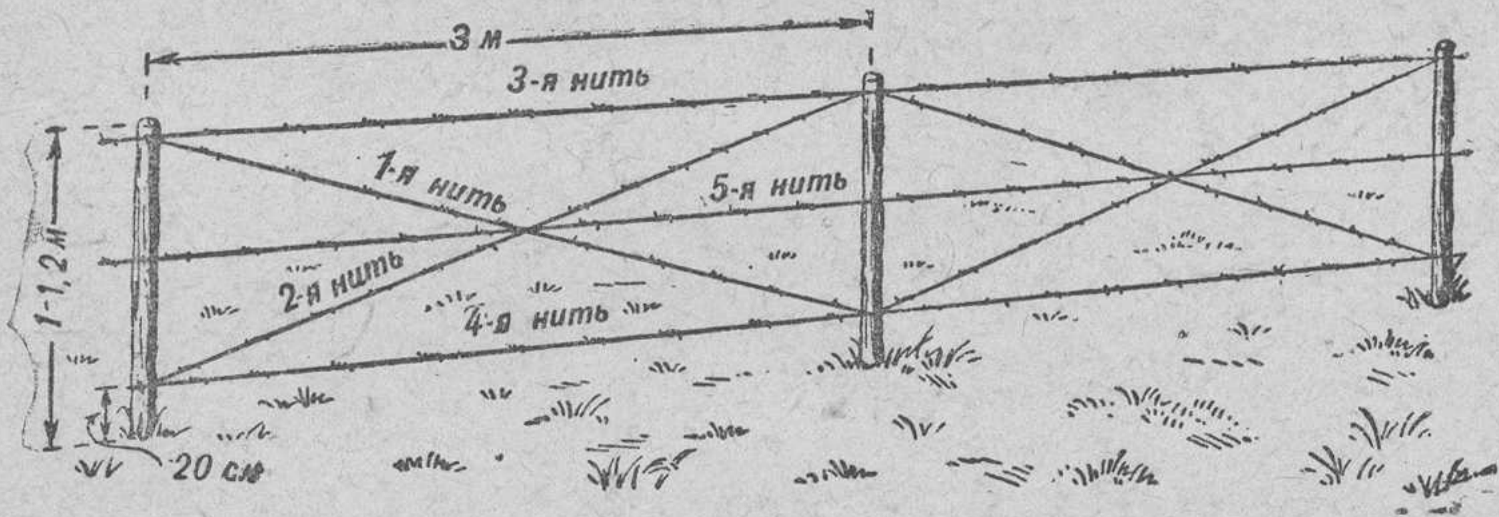
Рис. 93. Проволочный забор в пять нитей оплетки
