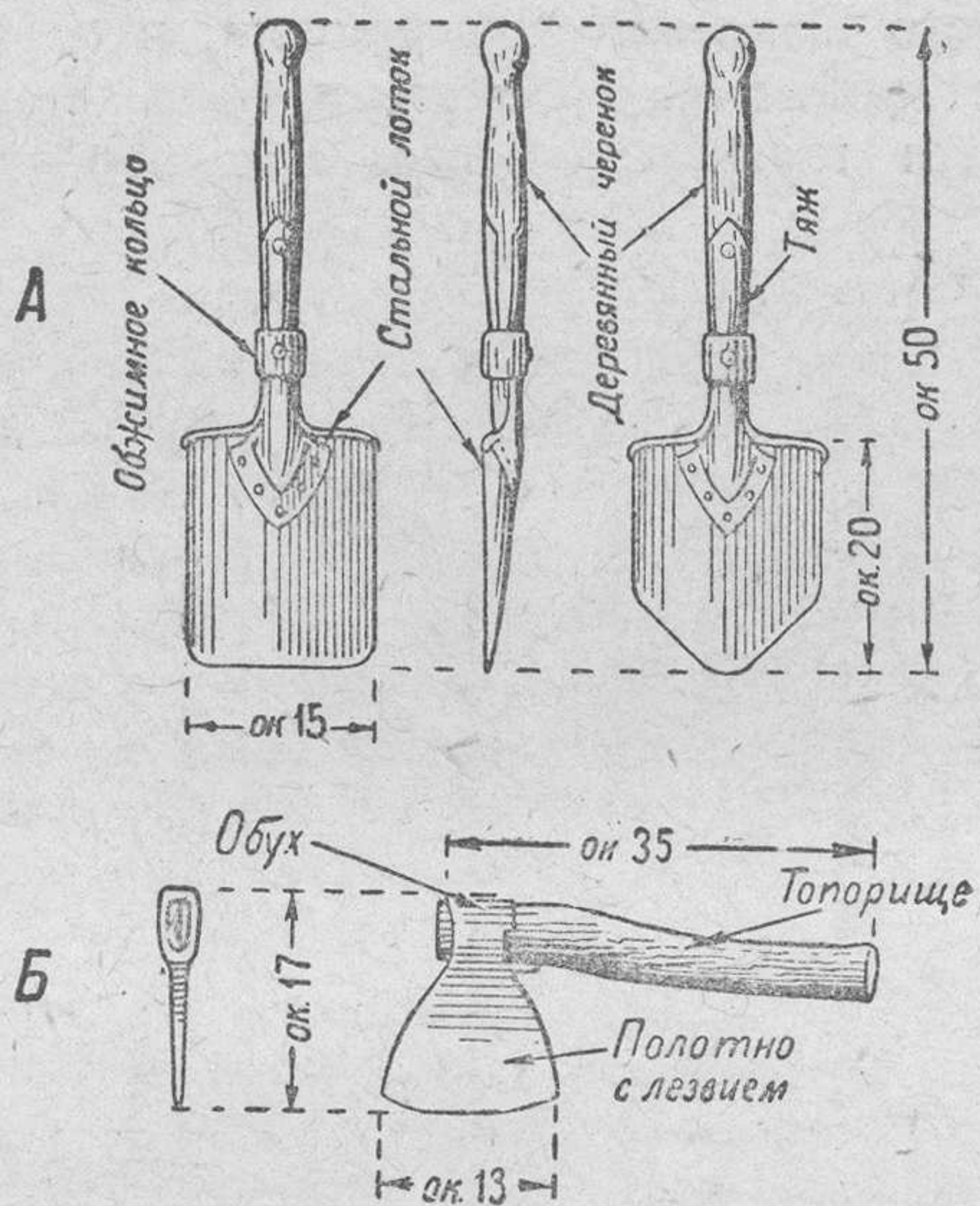
Рис. 7. Носимый шанцевый инструмент: А — малая лопата; Б — военный топор
