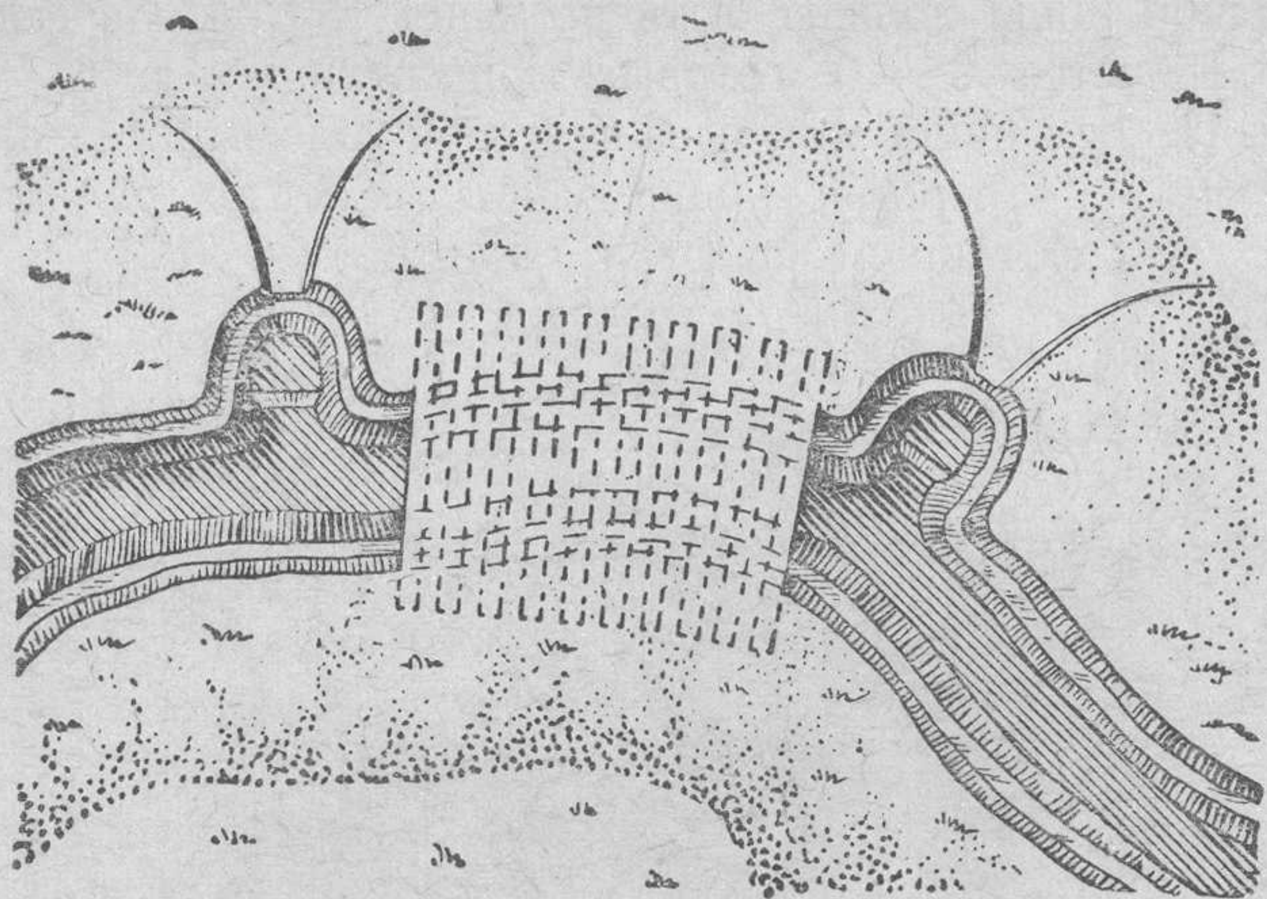
Рис. 55. Перекрытие над окопом
