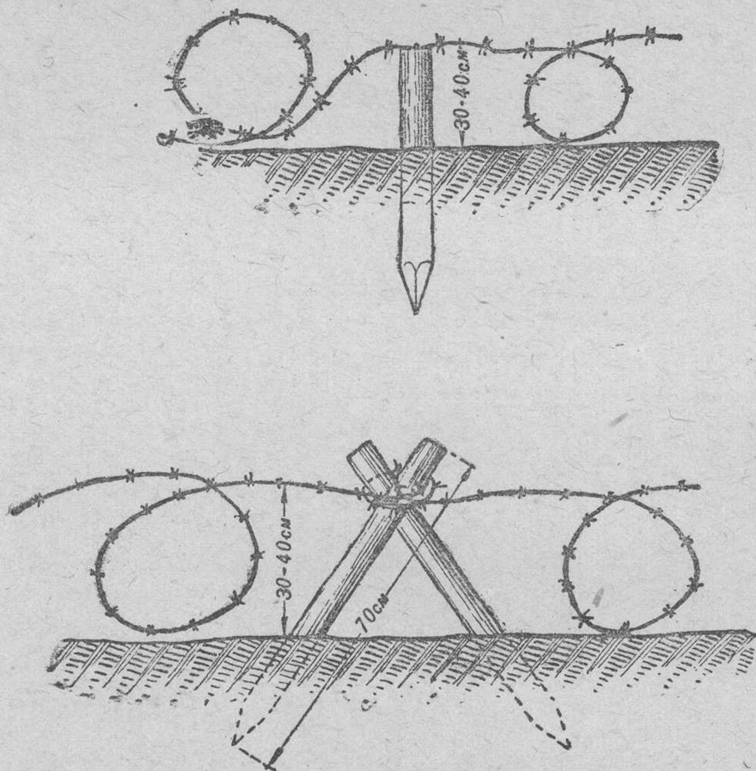
Рис. 89. Прикрепление проволоки к колышкам и козелкам
