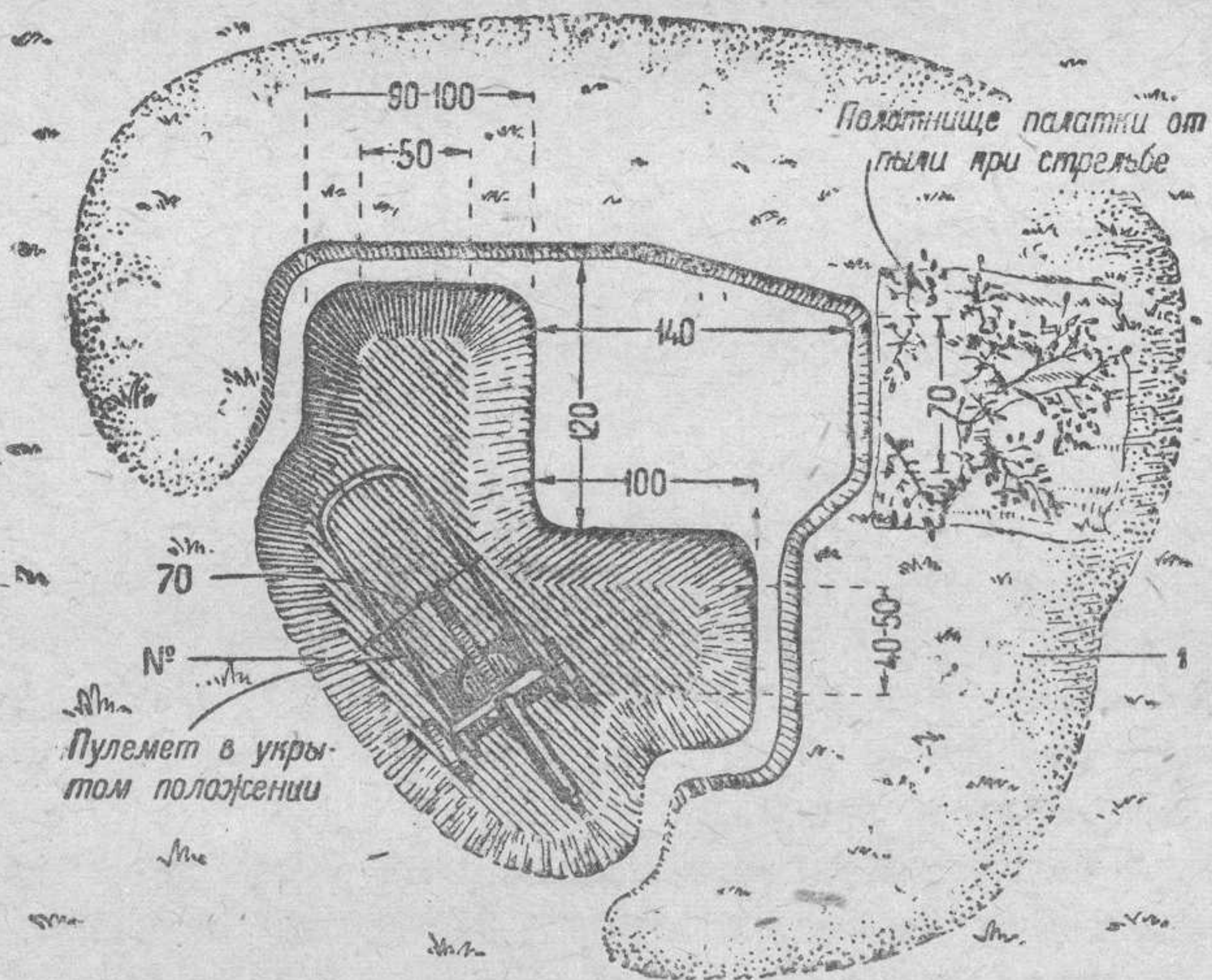
Рис. 27. Ячейка для ведения огня из станкового пулемета стоя Наводчик пулемета и его помощник отроют ячейку малыми лопатами и замаскируют ее за 1 час 45 минут
