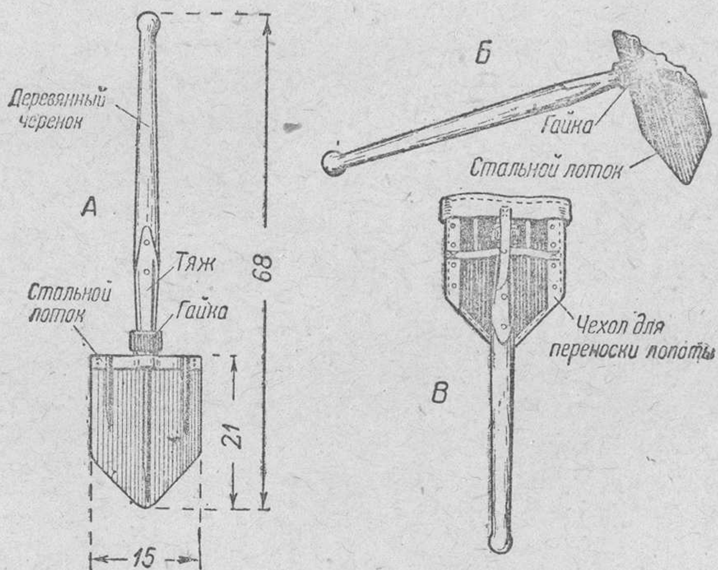
Рис. 7а. Немецкая пехотная лопата (трофейная): А — рабочее положение лопаты при отрывке; Б — положение лопаты при работе ею как мотыгой; В — положение лопаты при переноске
