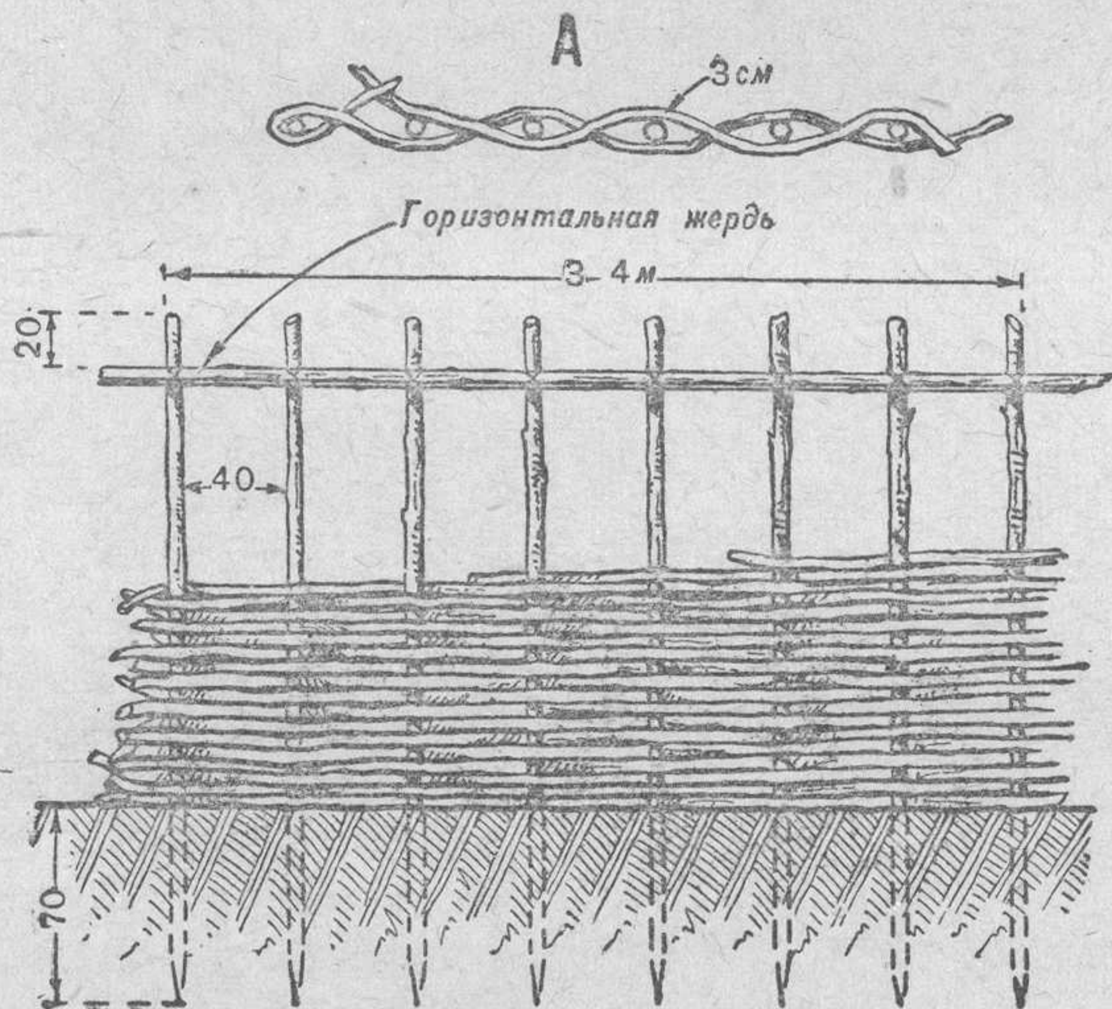
Рис. 64. Изготовление плетня:
