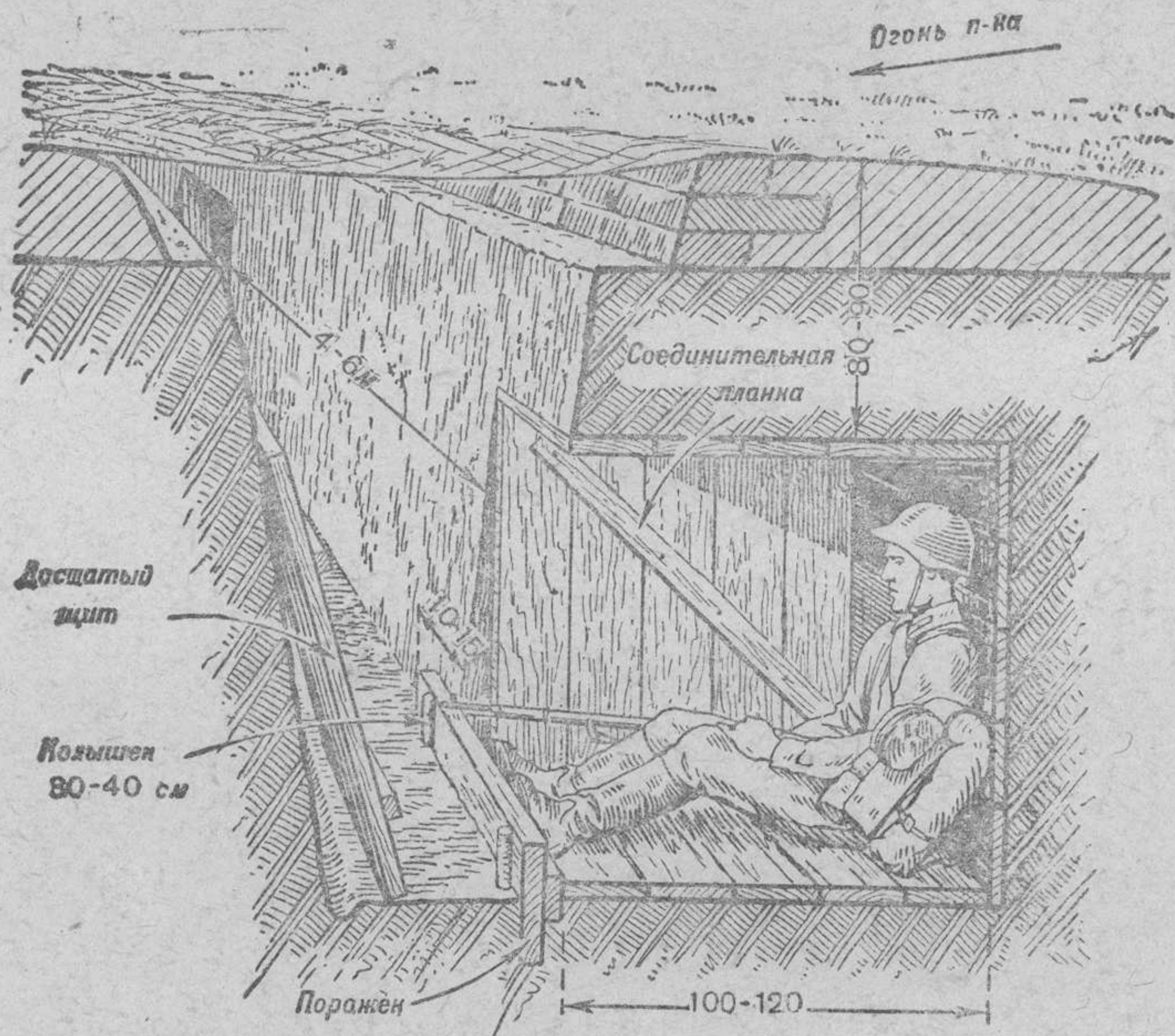
Рис. 52. Ниша из готовых дощатых рам для укрытия двух бойцов
