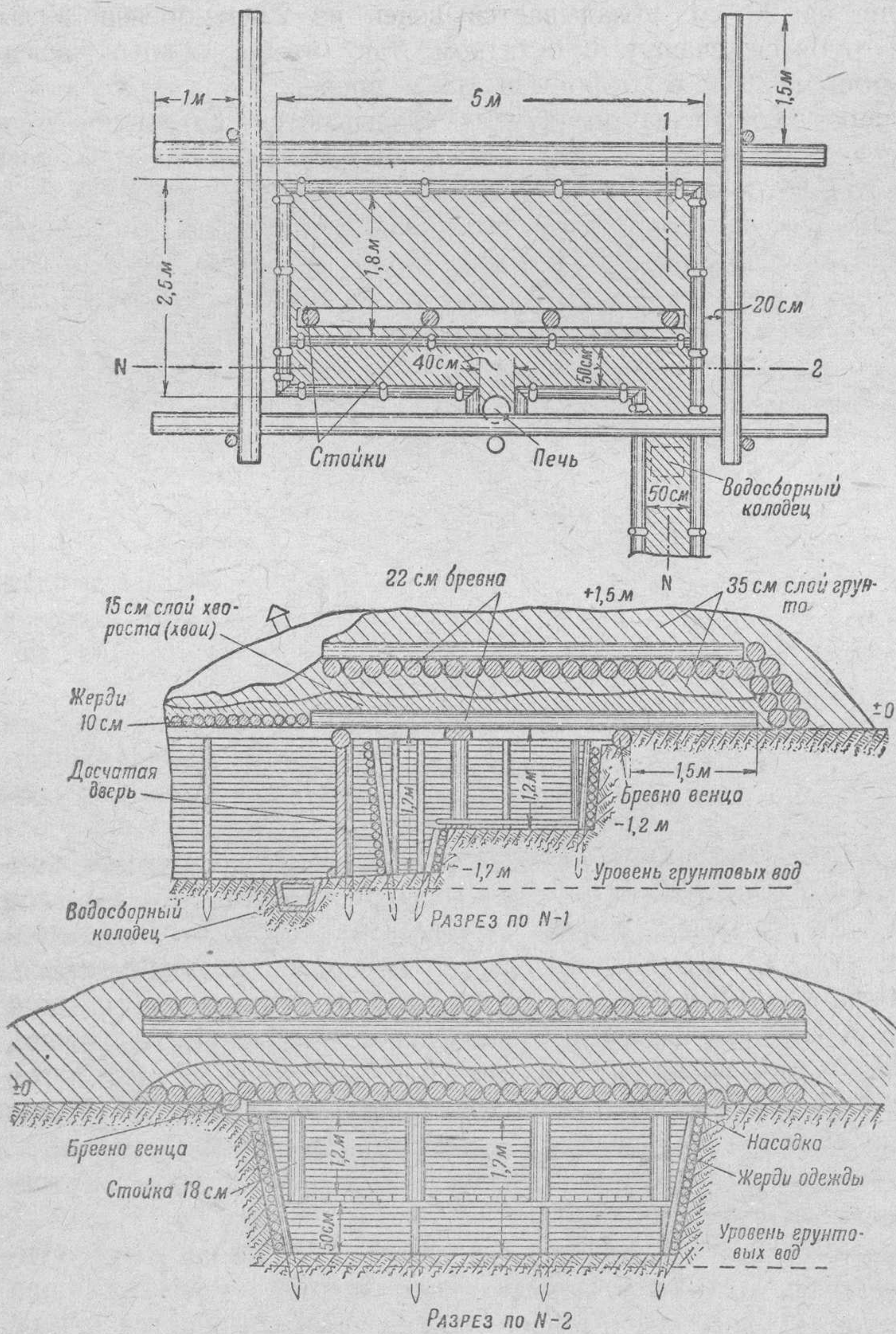
Рис. 81. Устройство землянки
