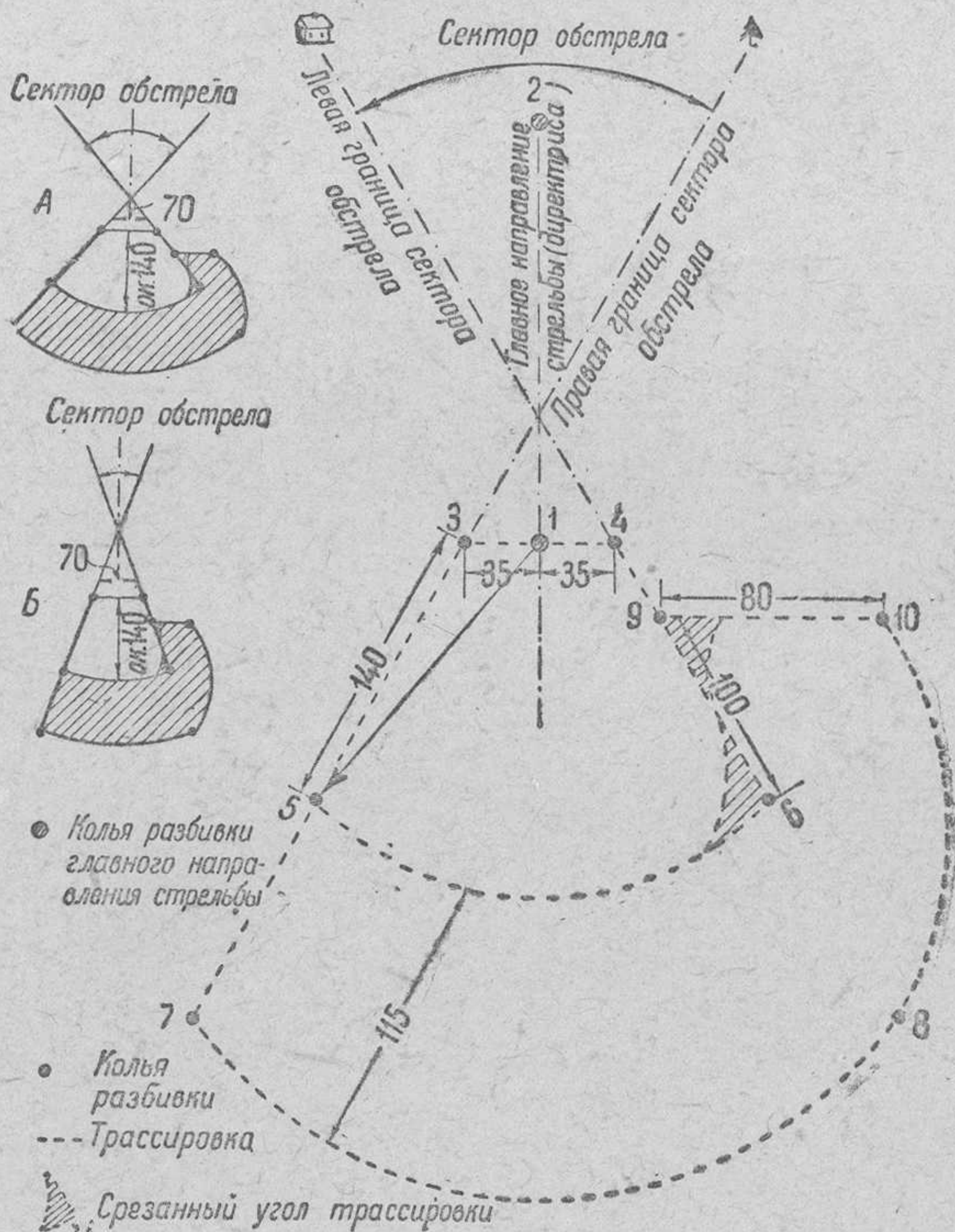
Рис. 35. Разбивка и трассировка пулеметной площадки в зависимости от заданного сектора обстрела:
