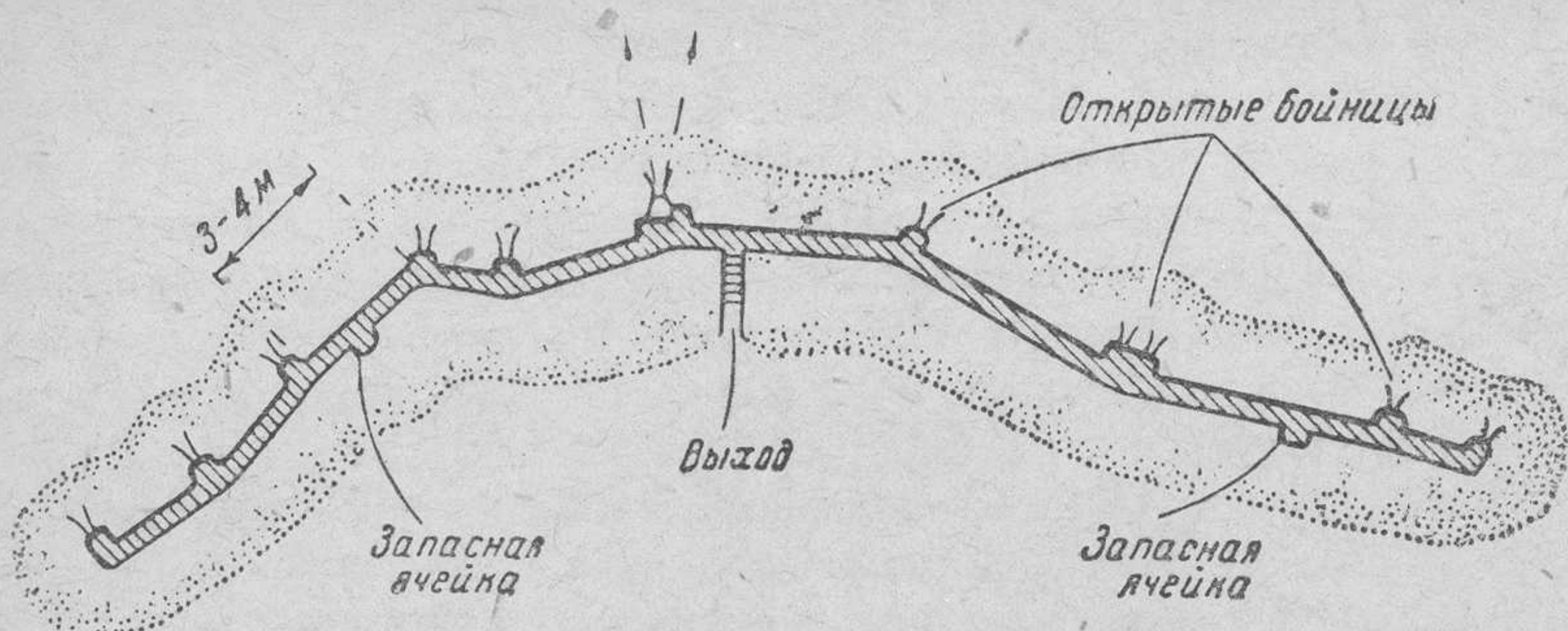
Рис. 3. Окоп на стрелковое отделение с заласными ячейками и выходом в тыл
