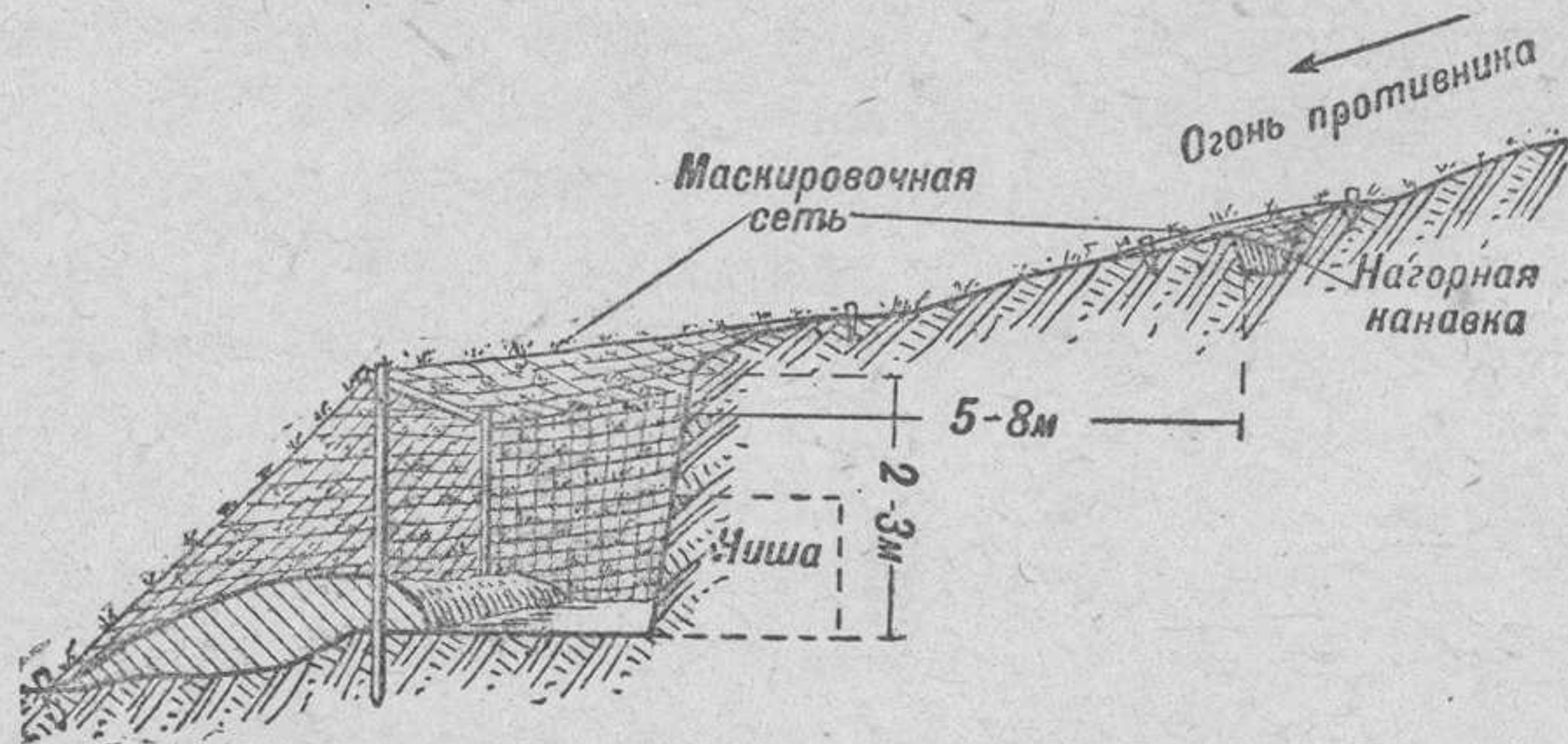
Рис. 79. Открытый заслон
