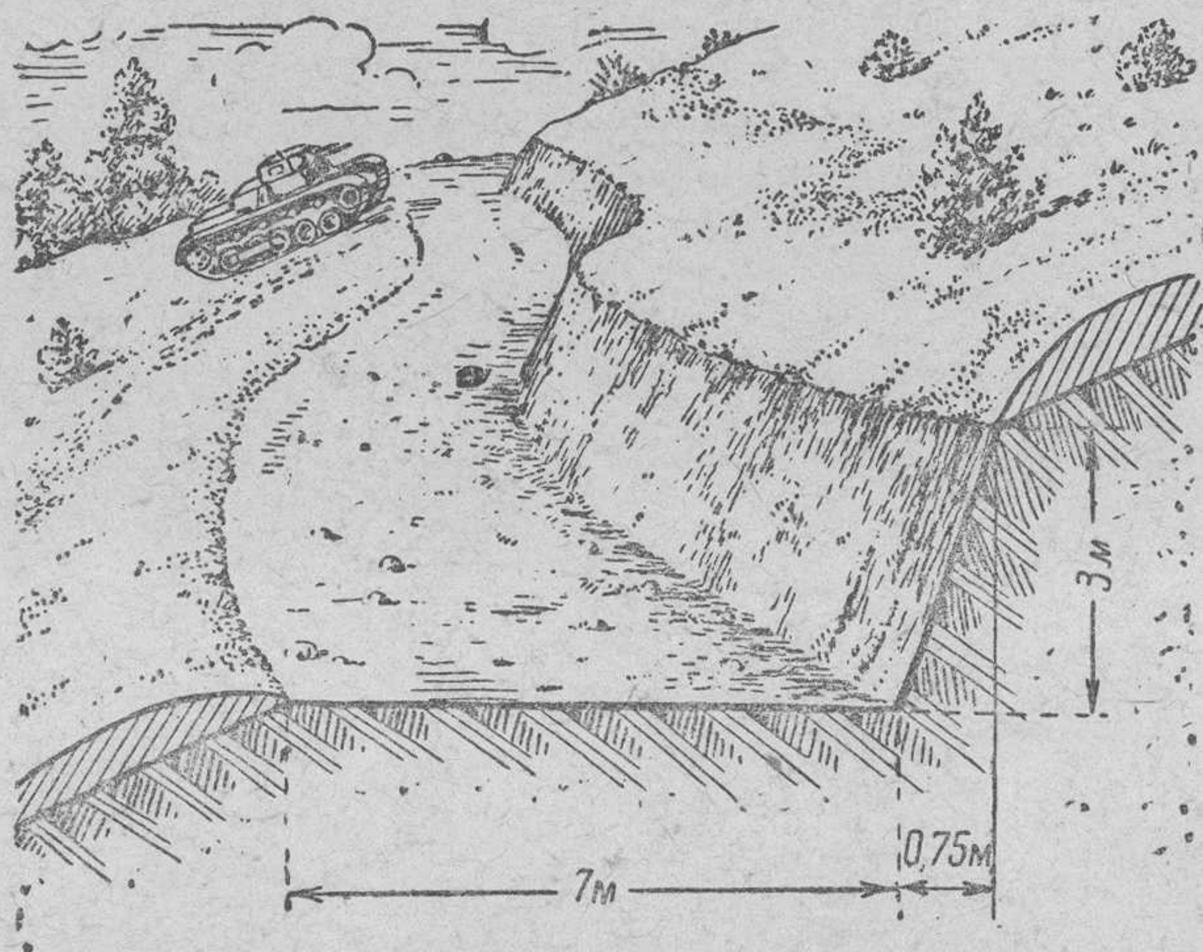
Рис. 110. Безбрустверный эскарп (без маскировки)
