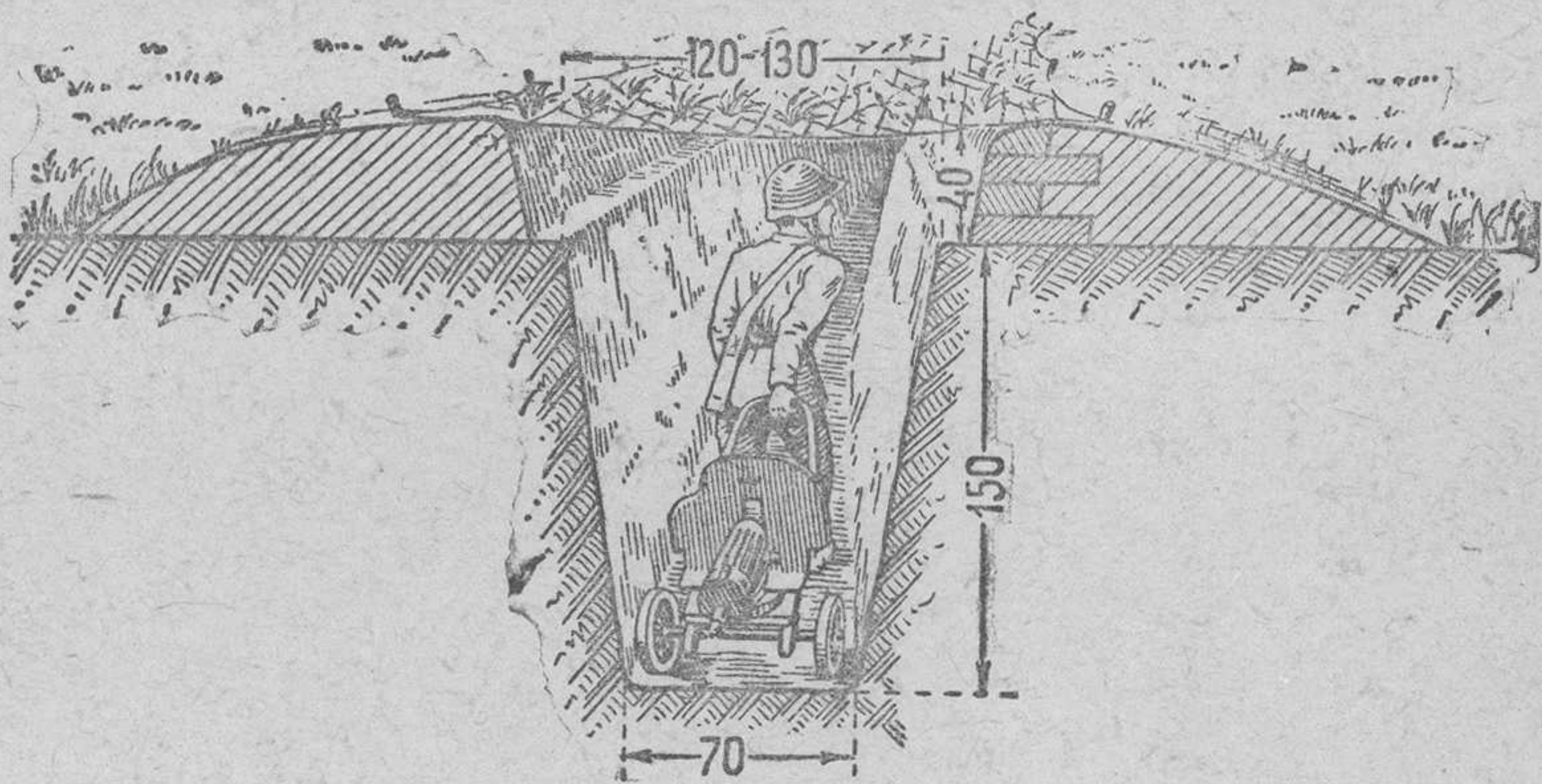
Рис. 34. Ход сообщения в пулеметном окопе
