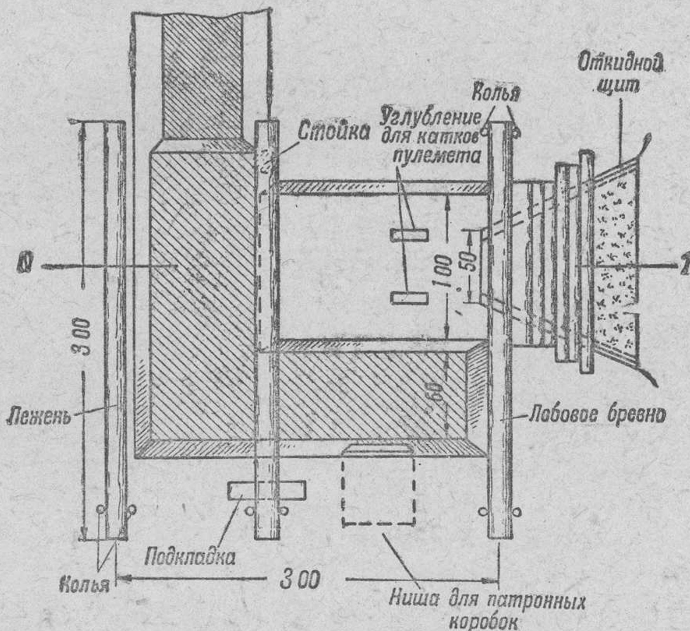
Рис. 40. Легкое блиндированное пулеметное гнездо
