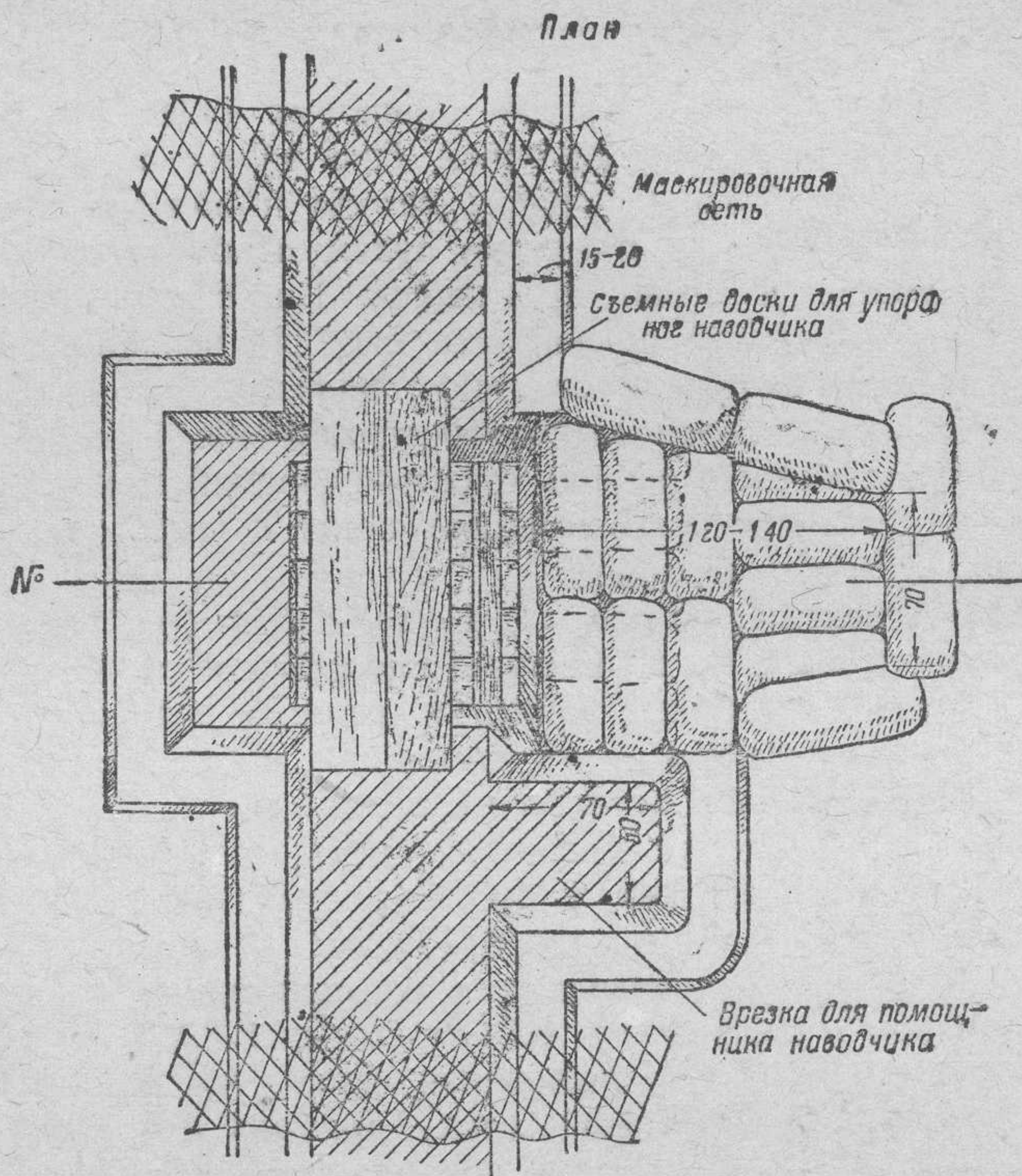
Рис. 39, А. Открытое пулеметное гнездо с укрытием-нишей (план)
