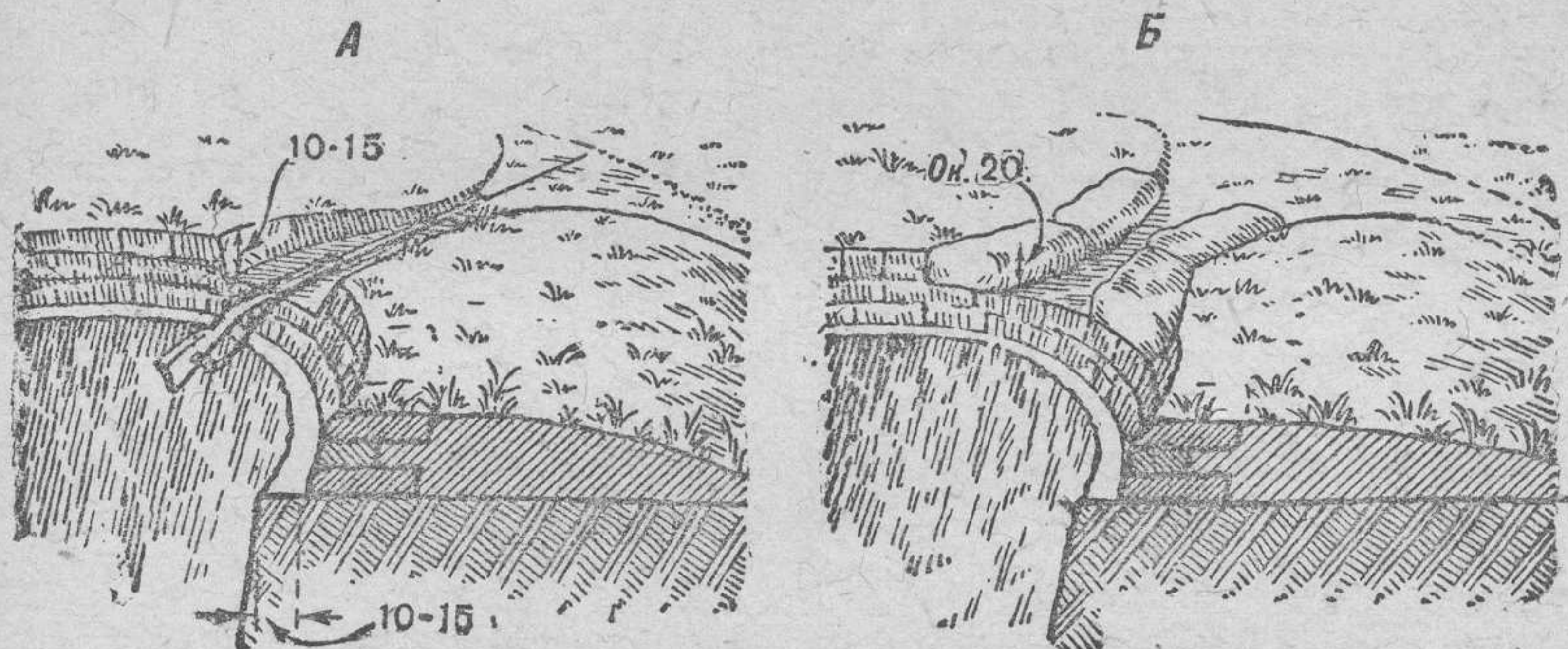
Рис. 42. Бойница из дернин и земляных мешков: А — бойница из дернин; Б — бойница из земляных мешков
