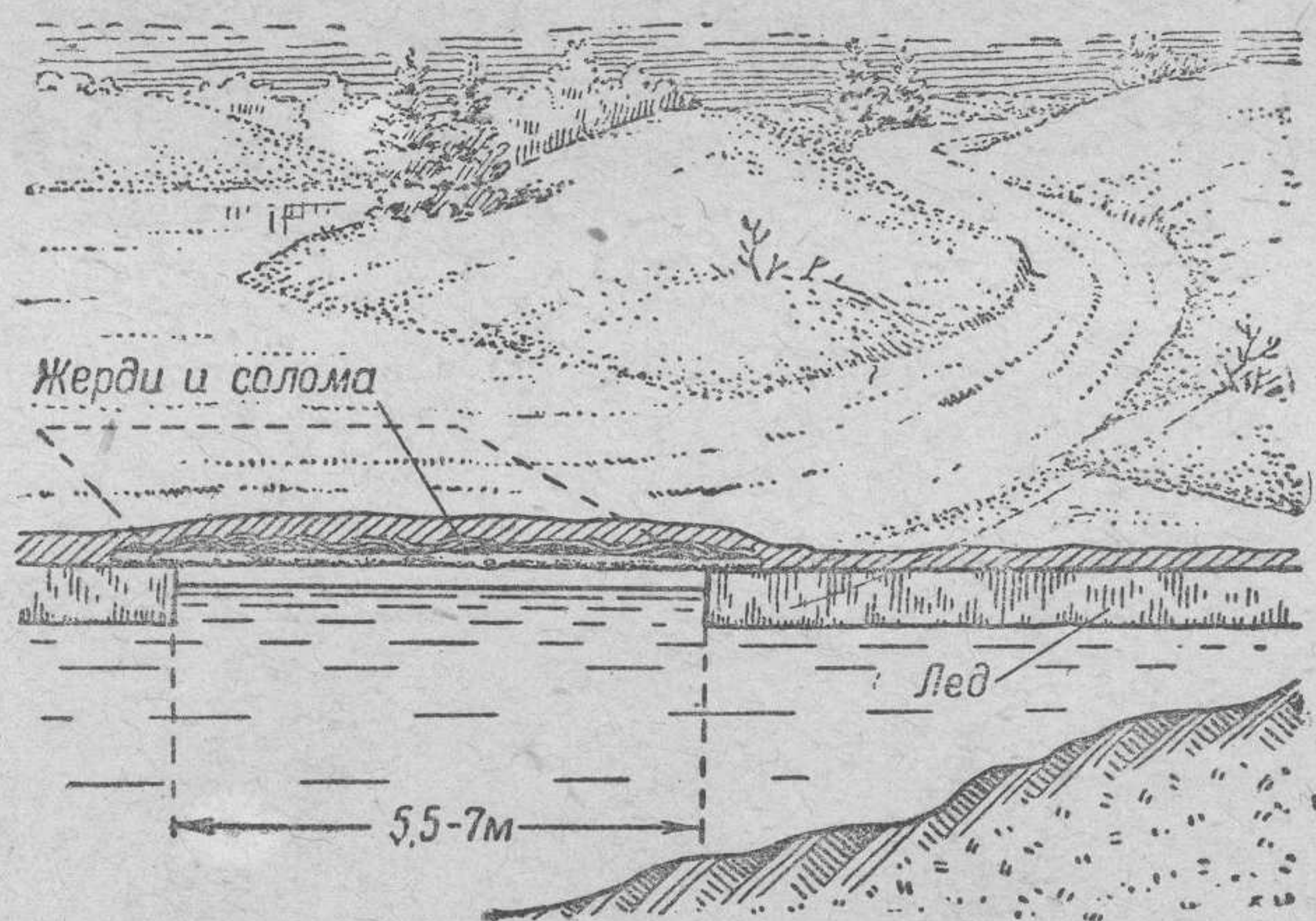
Рис. 119. Утепленная полынья-ловушка
