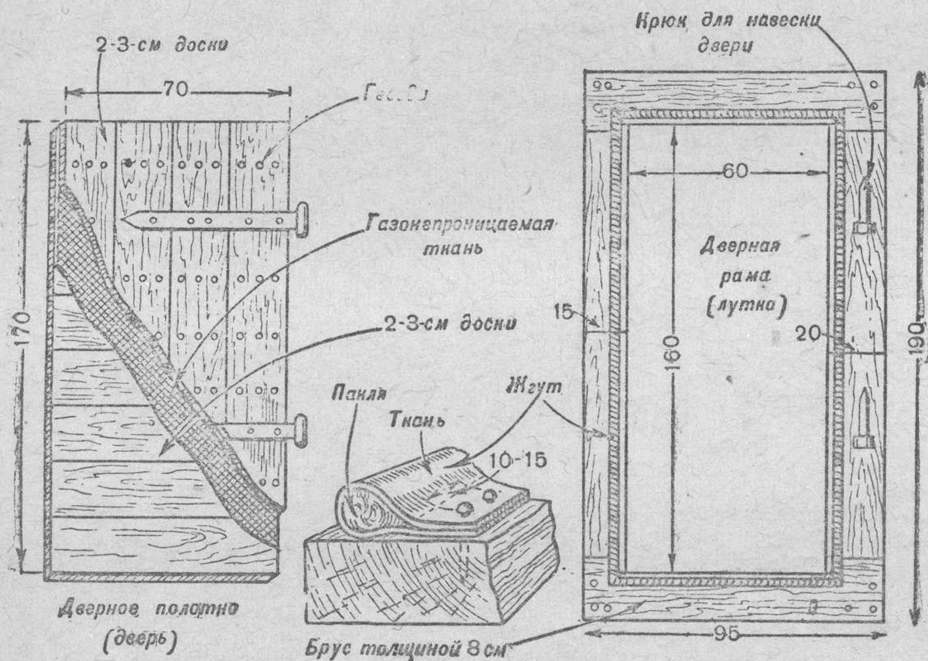
Рис. 84. Устройство герметической (газонепроницаемой) двери
