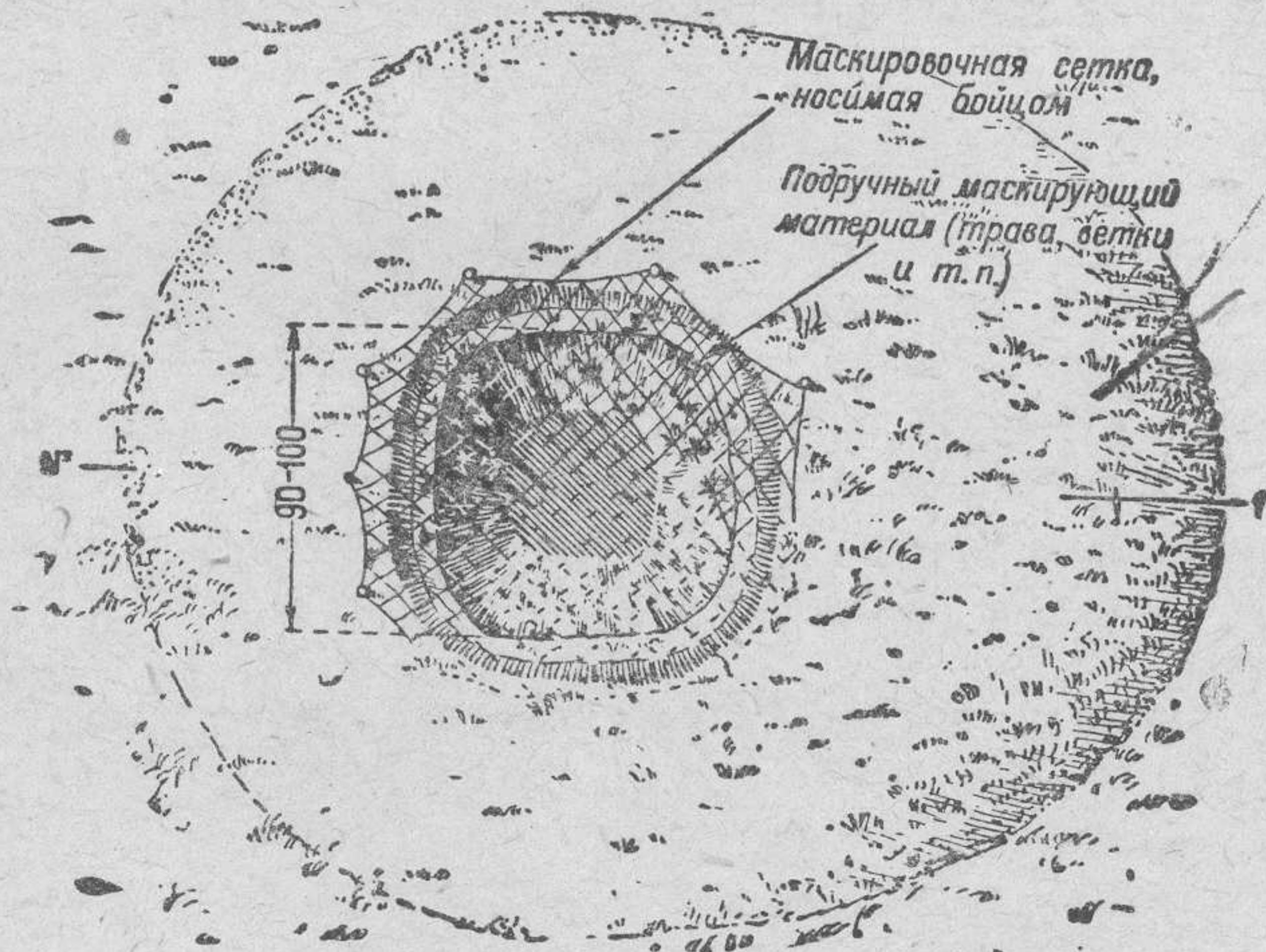
Рис. 26. Стрелковая ячейка для ведения огня стоя Боец отрывает такую ячейку малой лопатой и маскирует ее за 50—60 минут
