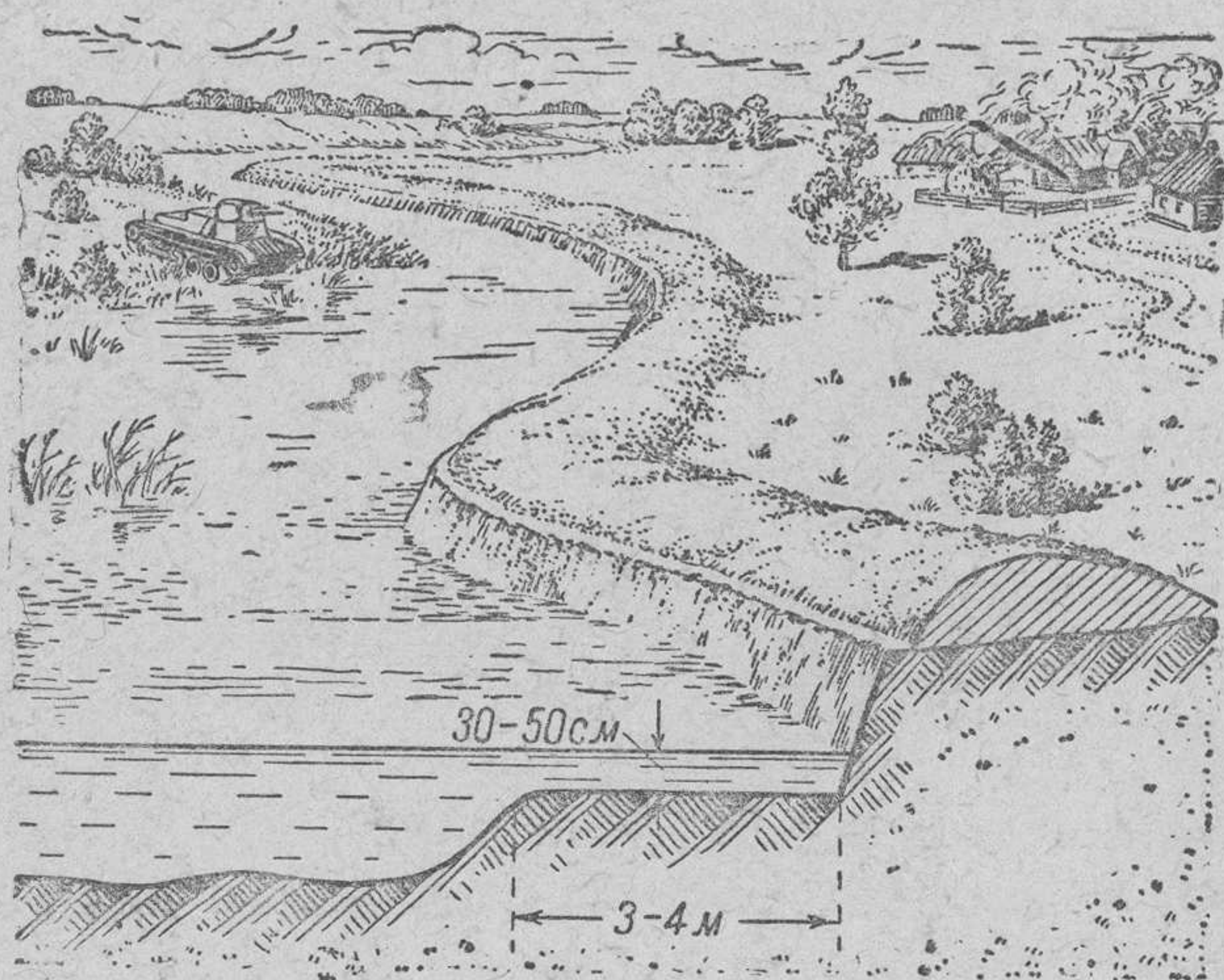
Рис. 111. Береговой эскарп
