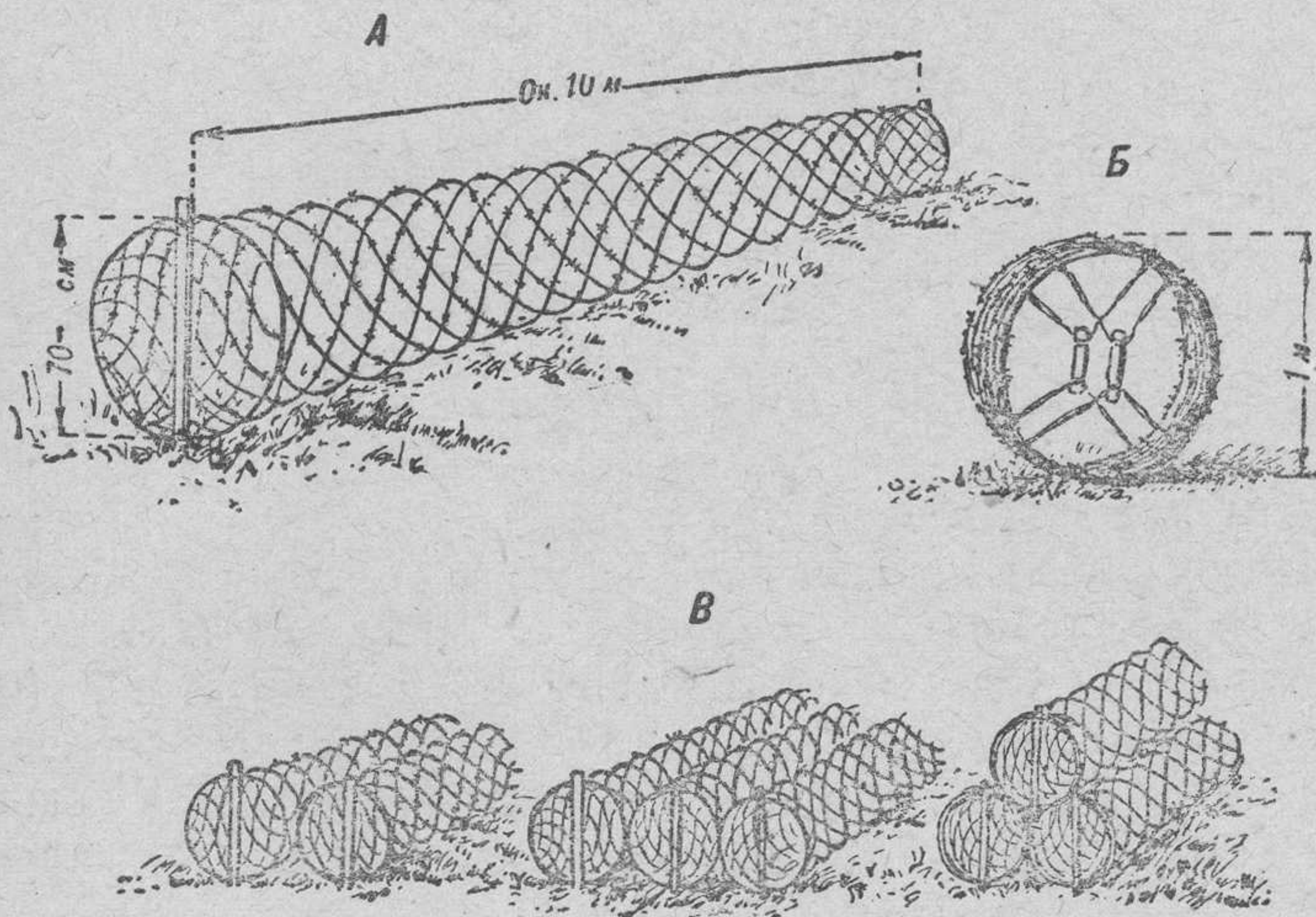
Рис. 105. Спираль Бруно:
