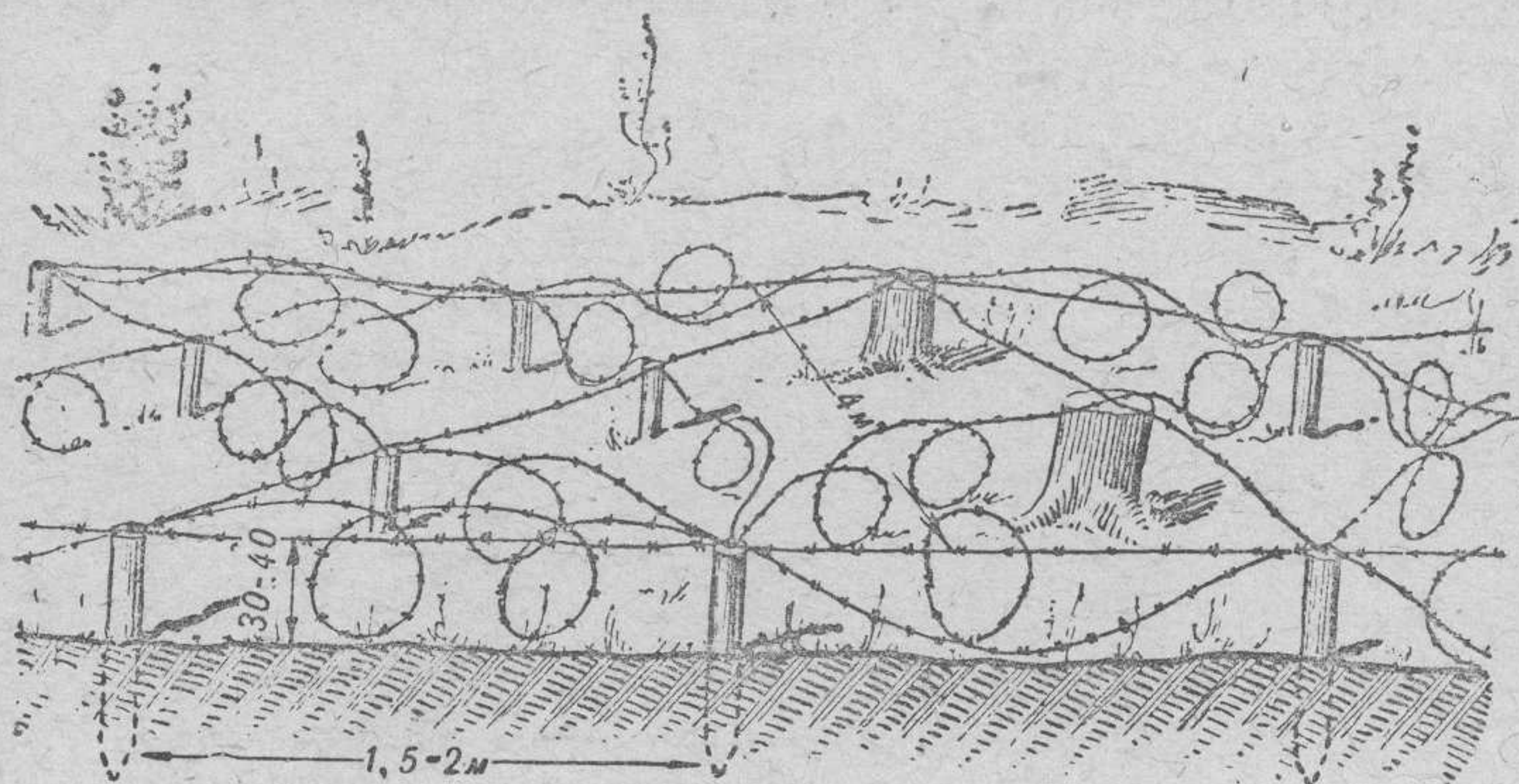
Рис. 90. Сеть на низких кольях («спотыкач»)
