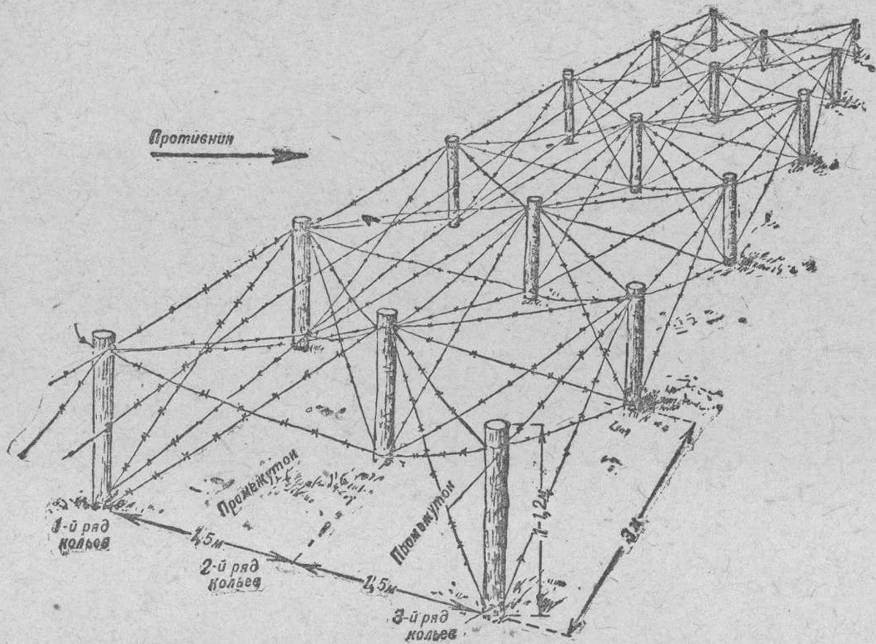
Рис. 92. Общий вид постоянной проволочной сети на деревянных кольях
