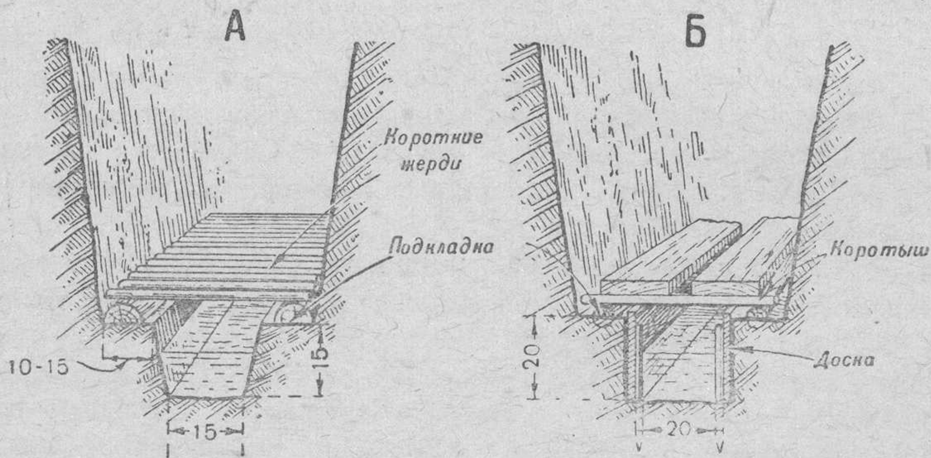
Рис. 68. Осушение дна окопа:
