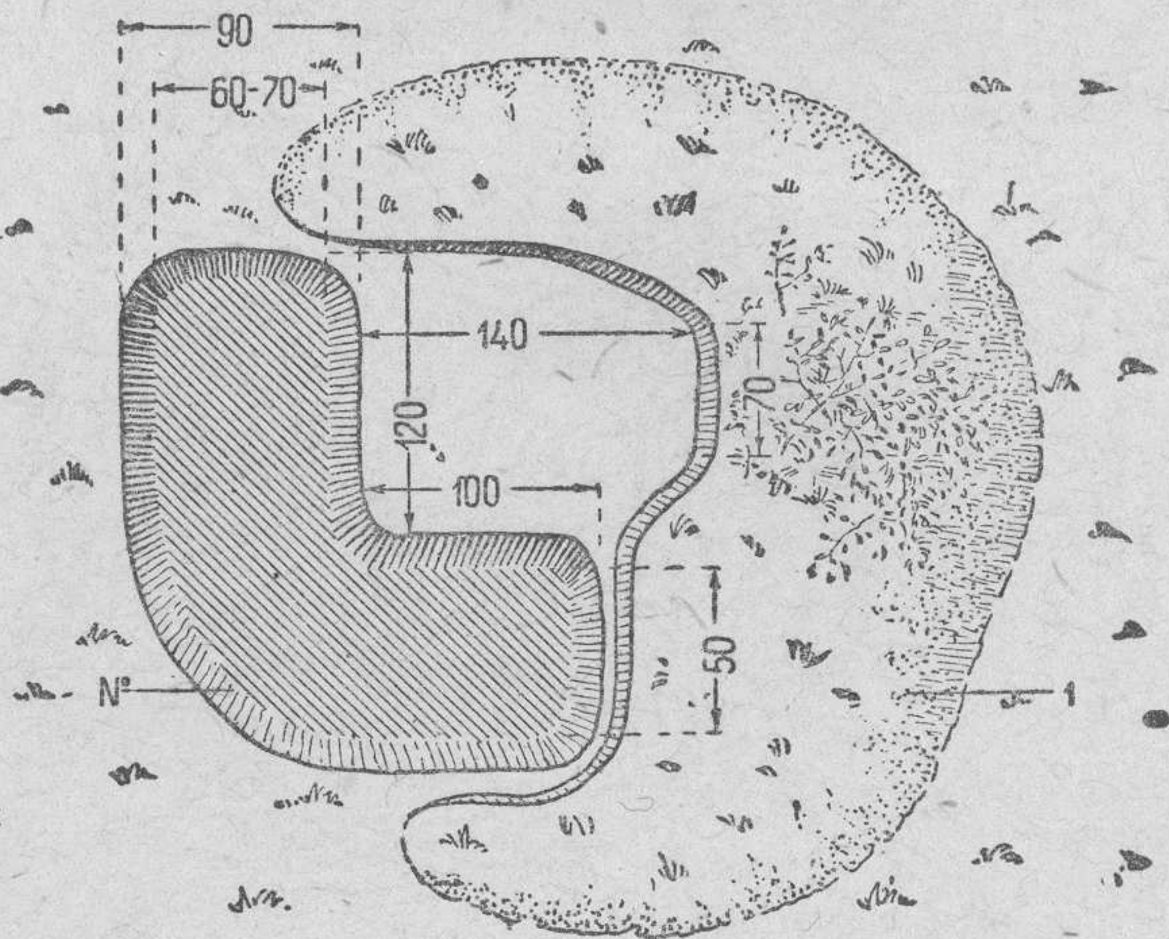
Рис. 25. Ячейка для ведения огня с колена из станкового пулемета Наводчик пулемета и его помощник малыми лопатами отроют ячейку и замаскируют ее за 30—40 минут
