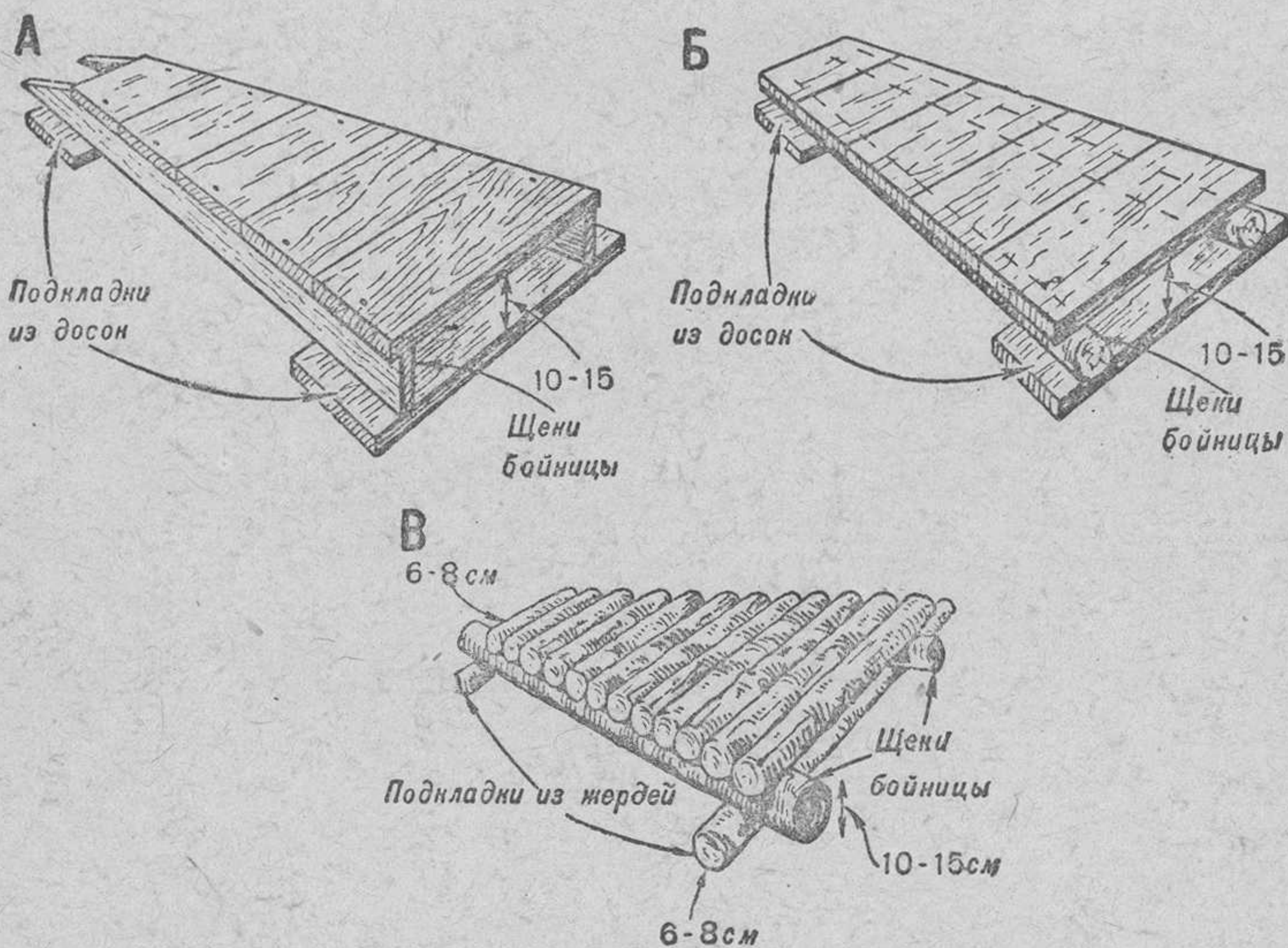
Рис. 44. Готовые бойницы:
