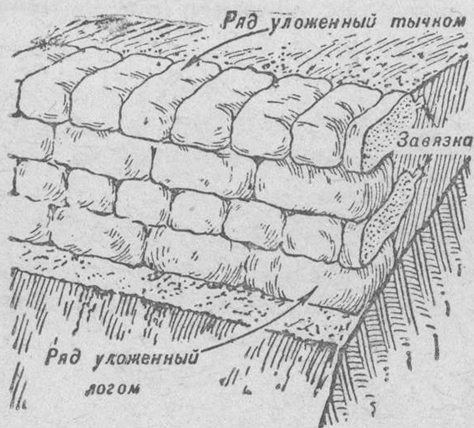
Рис. 65. Бруствер из земляных мешков
