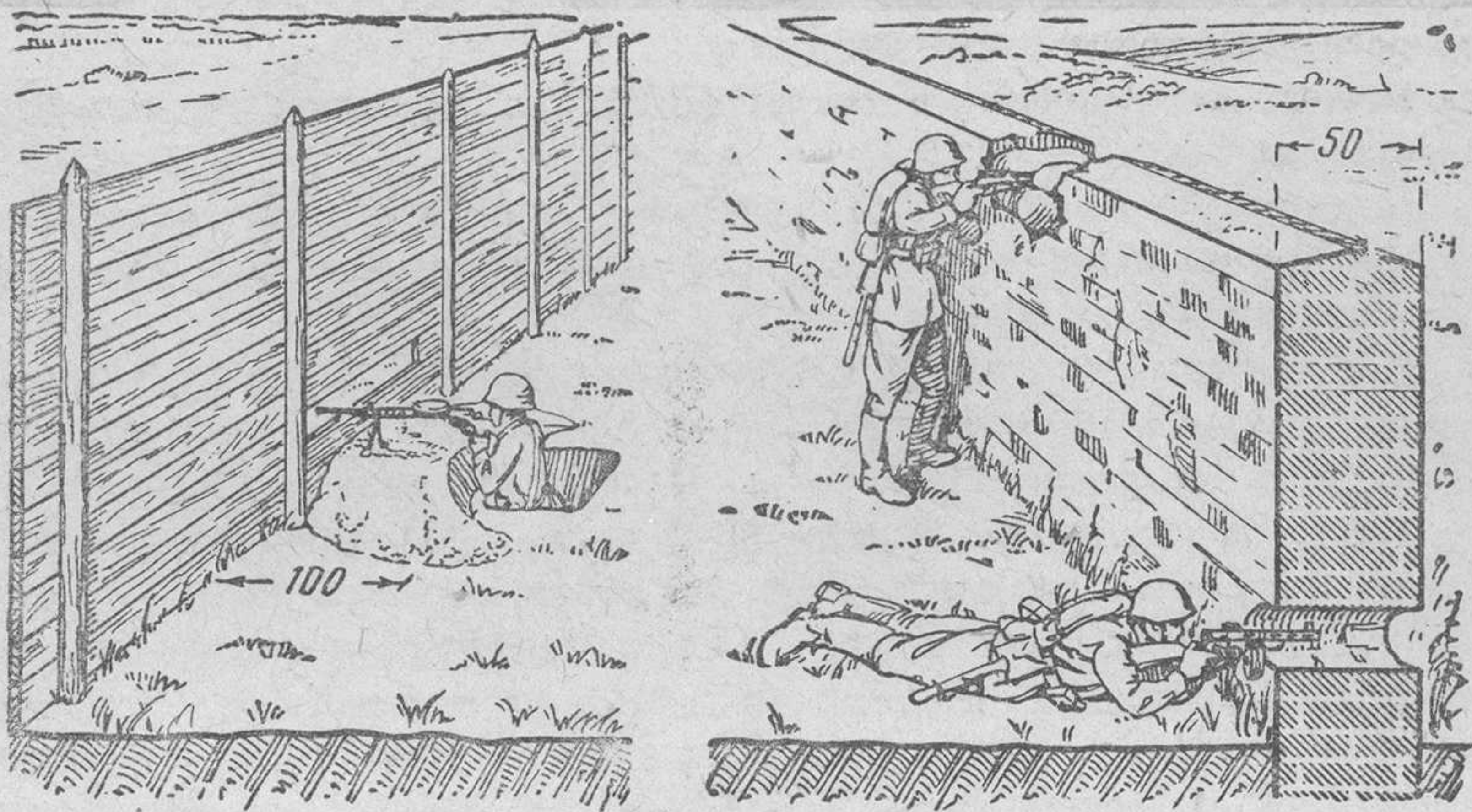
Рис. 73. Приспособление к обороне деревянного забора (слева) и каменной стенки (справа)
