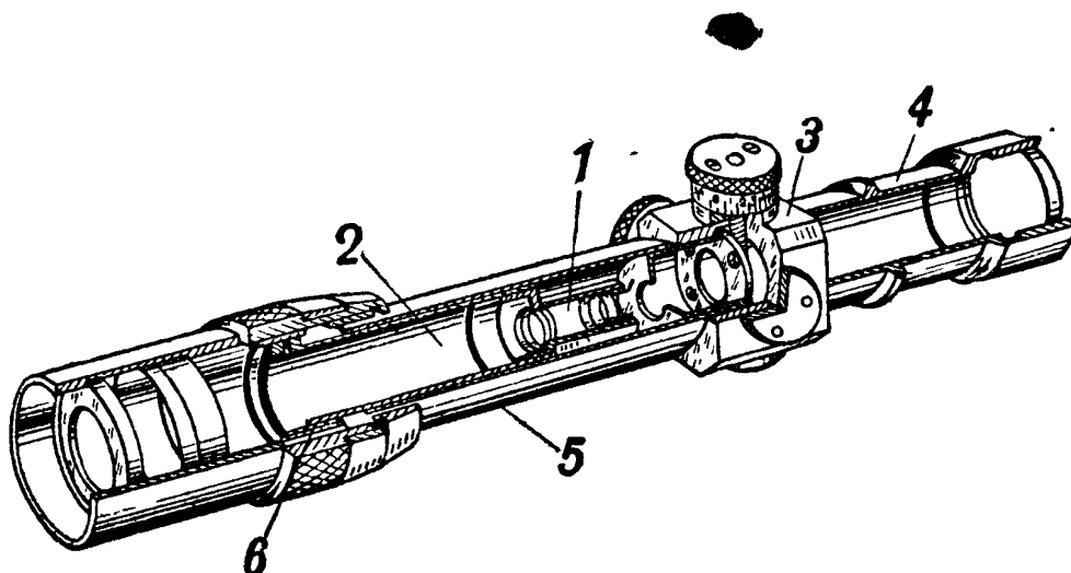
Рис. 91. Оптический прицел ПЕ в разрезе:
