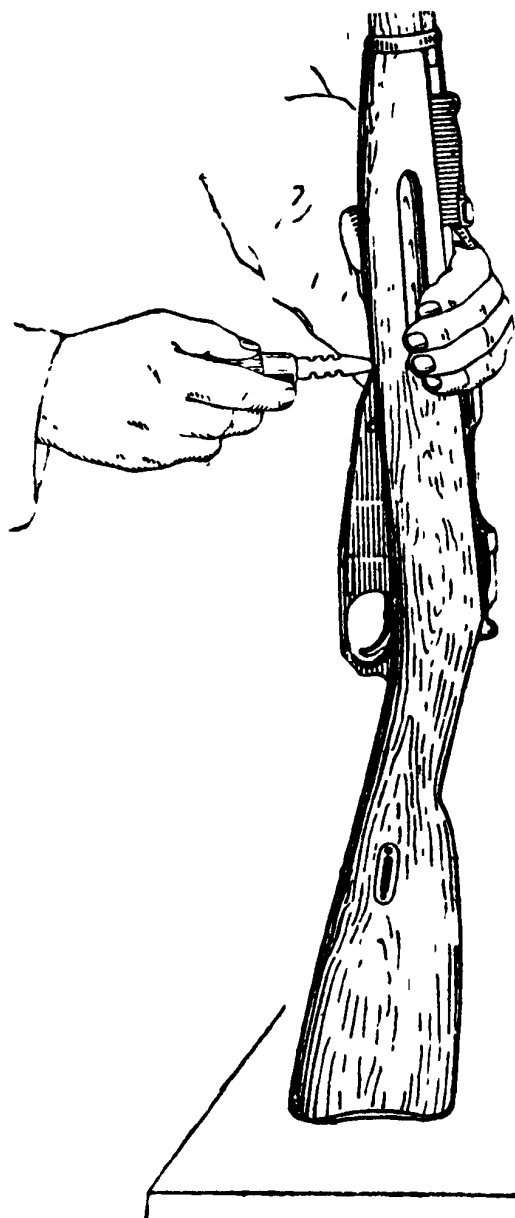
Рис. 52. Вывинчивание винта упора
