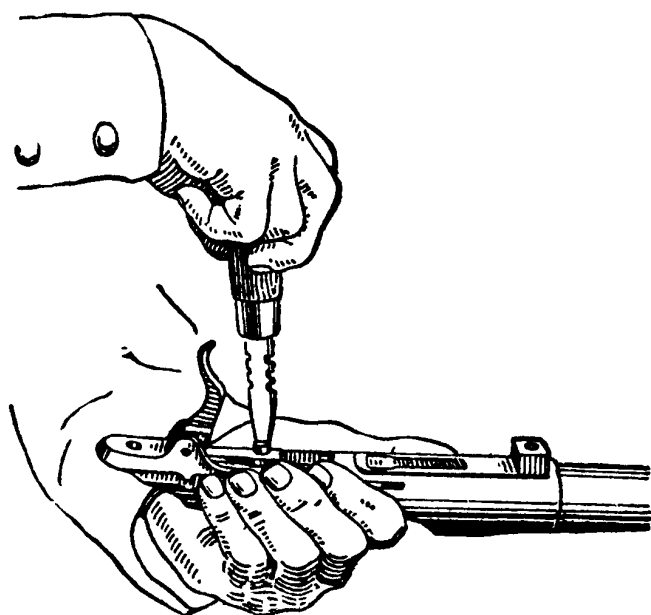
Рис. 54. Вывинчивание винта спусковой пружины
