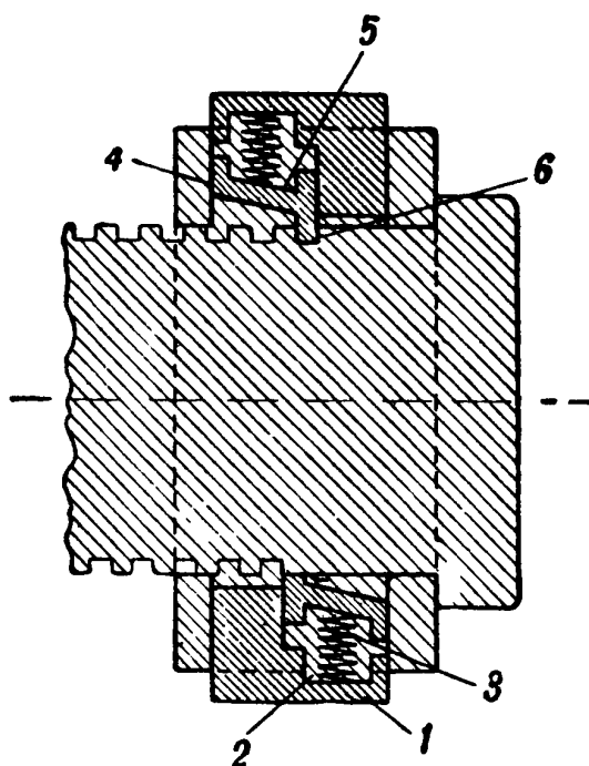
Рис. 9. Защелка прицельного хомутика:
