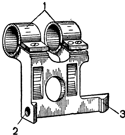
Рис. 95. Корпус кронштейна к оптическому прицелу ПУ:
