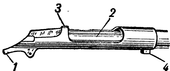
Рис. 3. Ствольная коробка: 1 — хвост; 2 — верхнее окно; 3 — пазы для обоймы; 4 — упор
