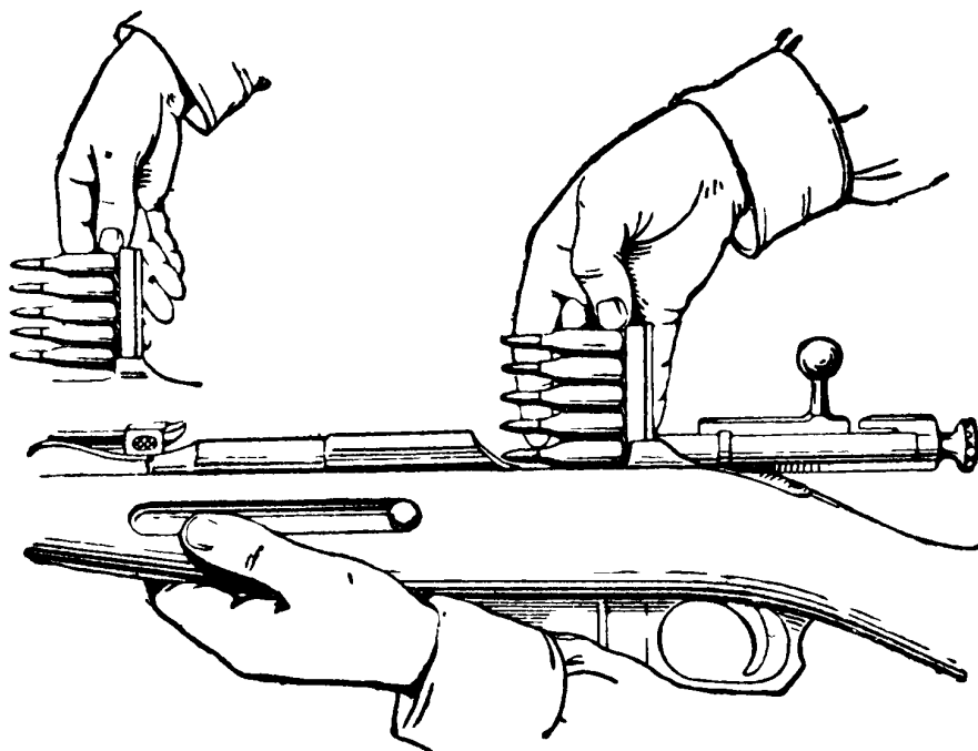
Рис. 63. Заряжание винтовки
