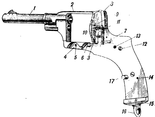
Рис. 8. Рамка с винченным стволом:
