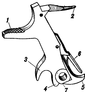
Рис. 12. Курок:
