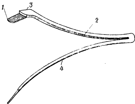
Рис. 13. Боевая пружина:
