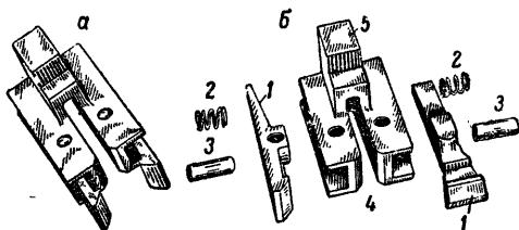
Рис. 14. Движок:
