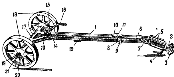
Рис. 19. Основание станка:
