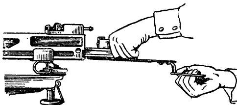
Рис. 26. Вынимание рамы с затвором из ствольной коробки
