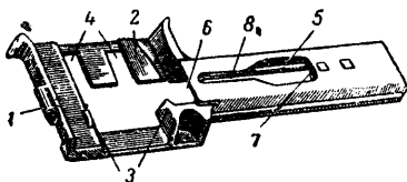
Рис. 12. Основание приемника:
