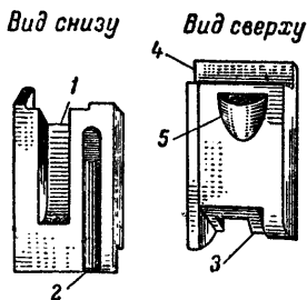
Рис. 17. Замыкатель ствола: 1 — выемка для сцепления со стволом; 2 — паз для прохода стопора; 3 — скос для пальцев подачи; 4 — срез для основания приемника; 5 — выемка для сдвигания замыкателя
