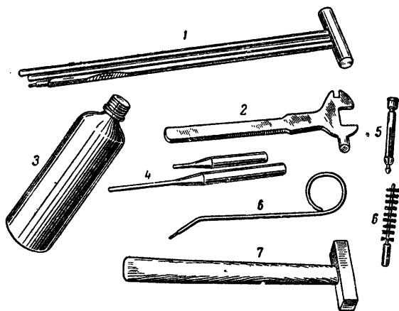
Рис. 22. Принадлежность:
