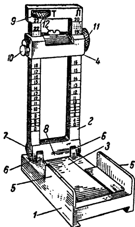
Рис. 7. Прицел:
