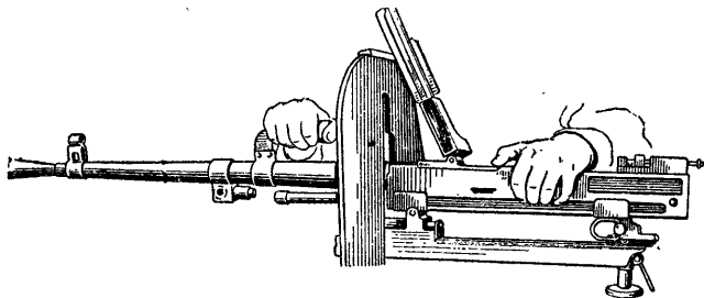
Рис. 27. Отделение ствола от ствольной коробки
