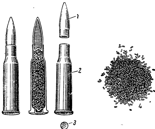
Рис. 23. Боевой патрон:
