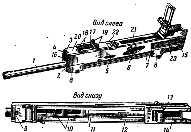
Рис. 6. Ствольная коробка:
