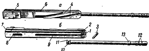
Рис. 8. Рама с поршнем:
