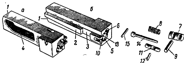
Рис. 9. Затвор:
