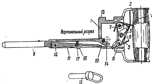
Рис. 11. Затыльник с направляющим стержнем возвратно-боевой пружины:
