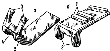
Рис. 16. Ползун с пальцами подачи:
