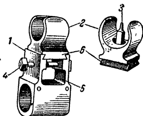
Рис. 5. Основание мушки с предохранителем и мушкой:
