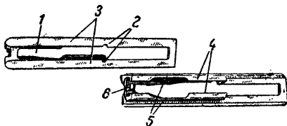
Рис. 13. Рамка приемника:
